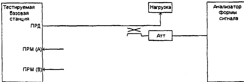
Рис.1.1.9. Схема измерения качества формы сигнала
