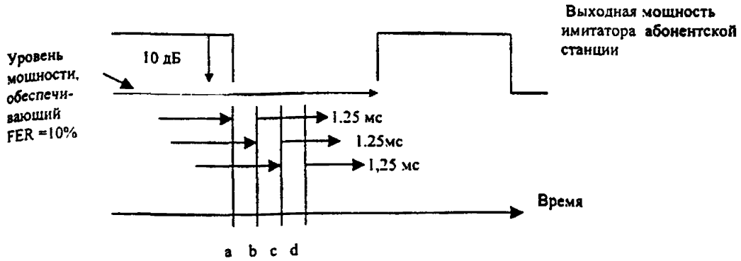
Рис.5.2.4-1 Интервалы команд увеличения мощности АС
