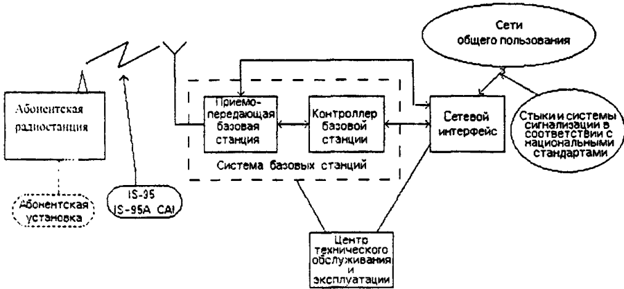
Рис.3. Конфигурация системы радиодоступа с CDMA
