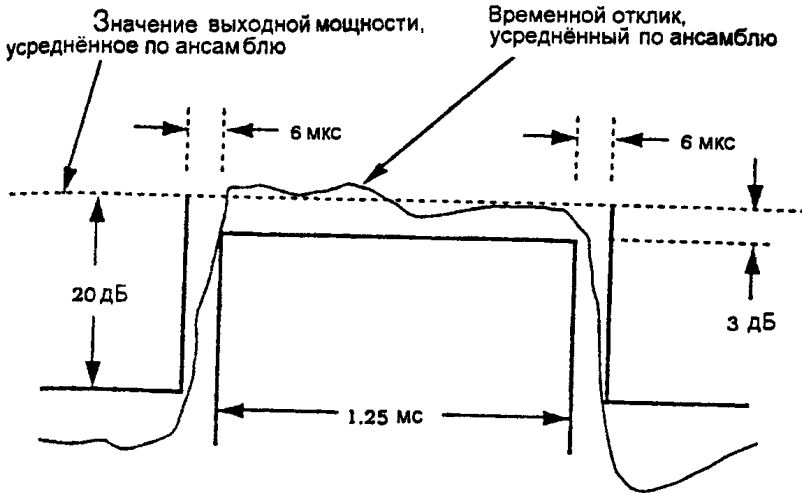
Рис.4.2.4.7. Шаблон огибающей мощности передатчика.
