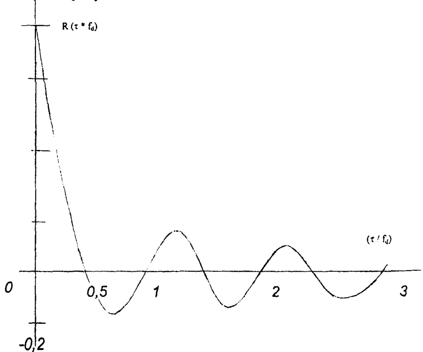
Рис.1.2.1. Функция автокорреляции фазы
