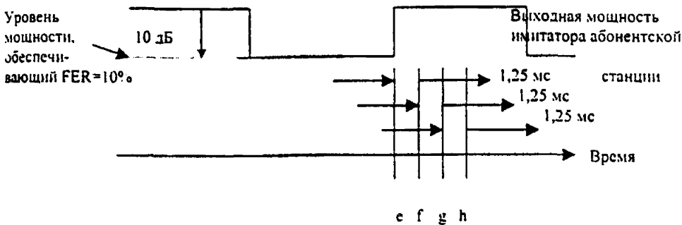
Рис.5.2.4-2 Интервалы команд уменьшения мощности АС
