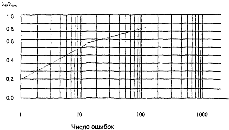
Рис. 1 Зависимость допустимого значения \lambda_N/\lambda_{lim} от числа ошибок K для доверительной вероятности 95%
