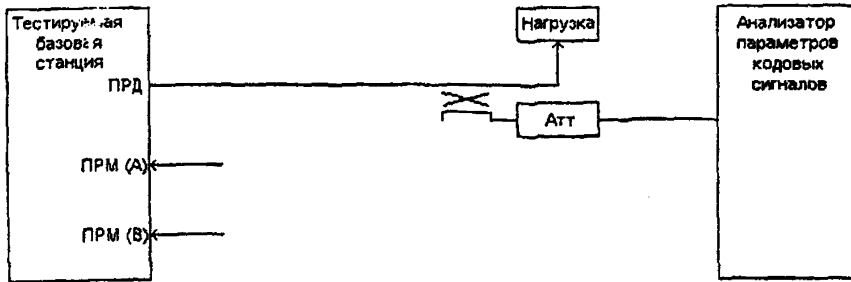
Рис.1.1.10. Схема измерения параметров кодовых сигналов
