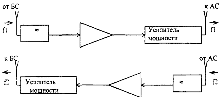
Рис. 6.1. Структурная схема немодулирующего ретранслятора
