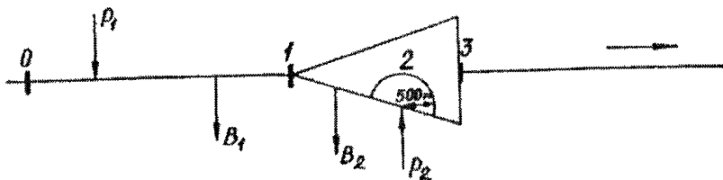
Рис. П 2.1. Линейная схема участка бассейна реки:
