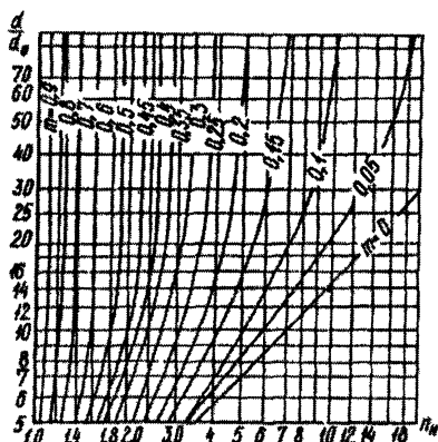
Рис.3.2. Номограмма для определения начального разбавления в потоке
