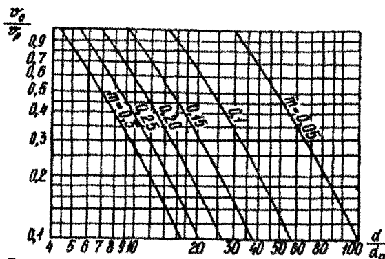
Рис.3.1. Номограмма для определения диаметра струи в расчетном сечении
