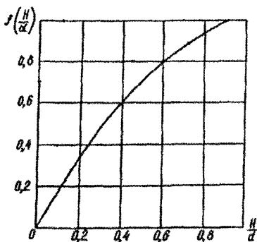
Рис.3.3. Номограмма для определения поправочного коэффициента
