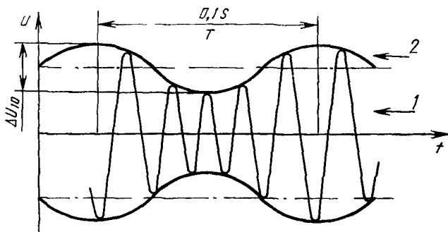
1 — постоянная частота сети 50 Гц; 2 — синусоидальное колебание напряжения
