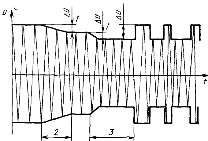
1 — изменения напряжения; 2 — продолжительность изменения; 3 — интервал изменения напряжения
