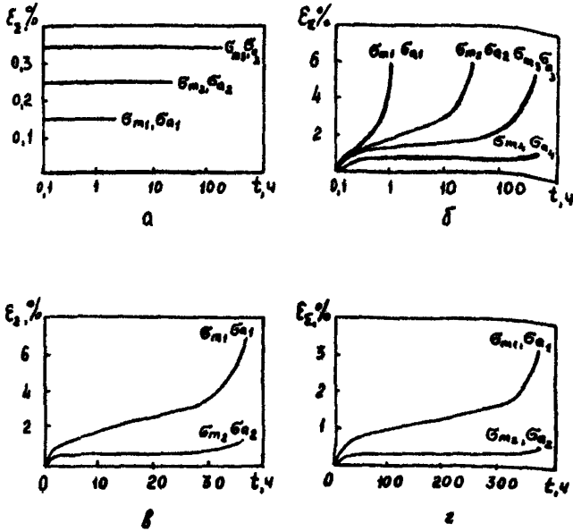
Рис.5. Характерные типы диаграмм ползучести при различных режимах силового и температурного воздействия:
