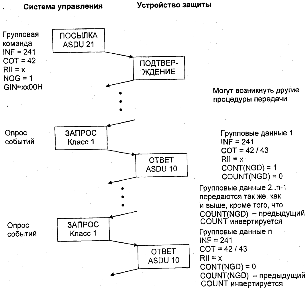
Рисунок 14 — Чтение значений или атрибутов всех элементов в одной группе
