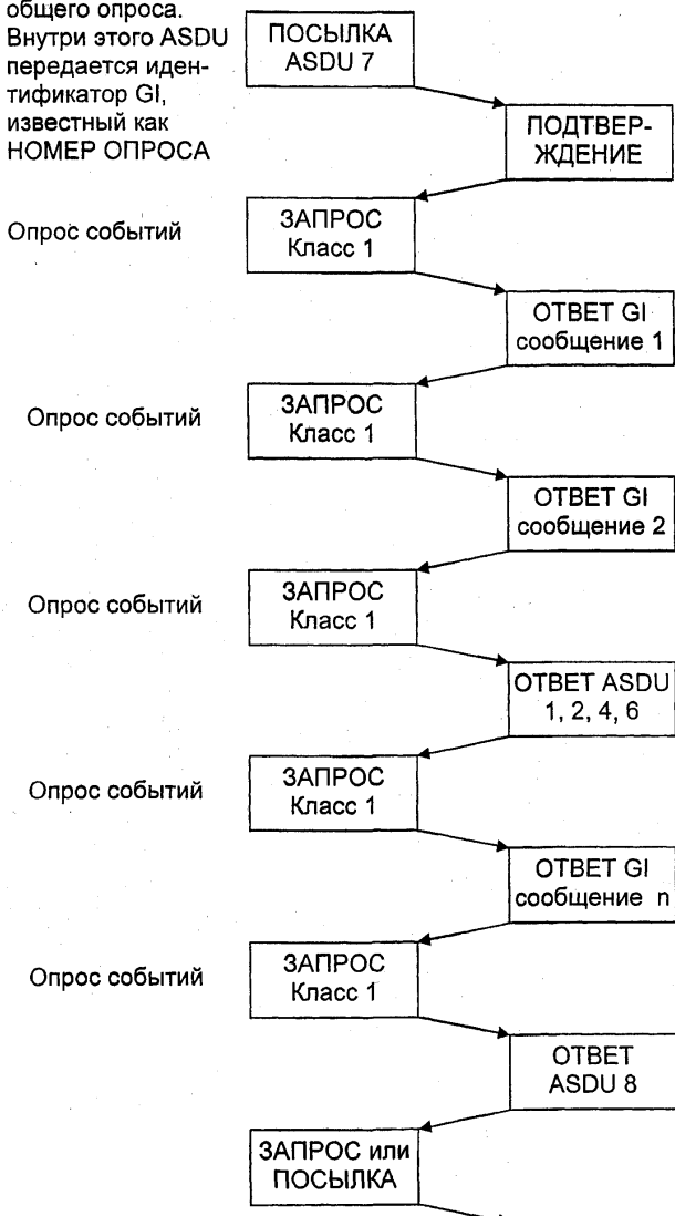
Рисунок 6 — Общий опрос
