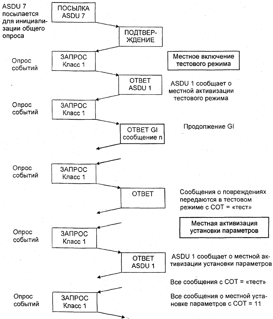
Рисунок 8 — Тестовый режим (лист 1)
