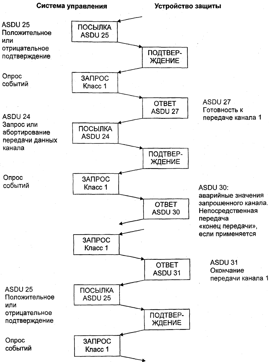
Рисунок 10 — Передача данных о нарушениях (лист 3)
