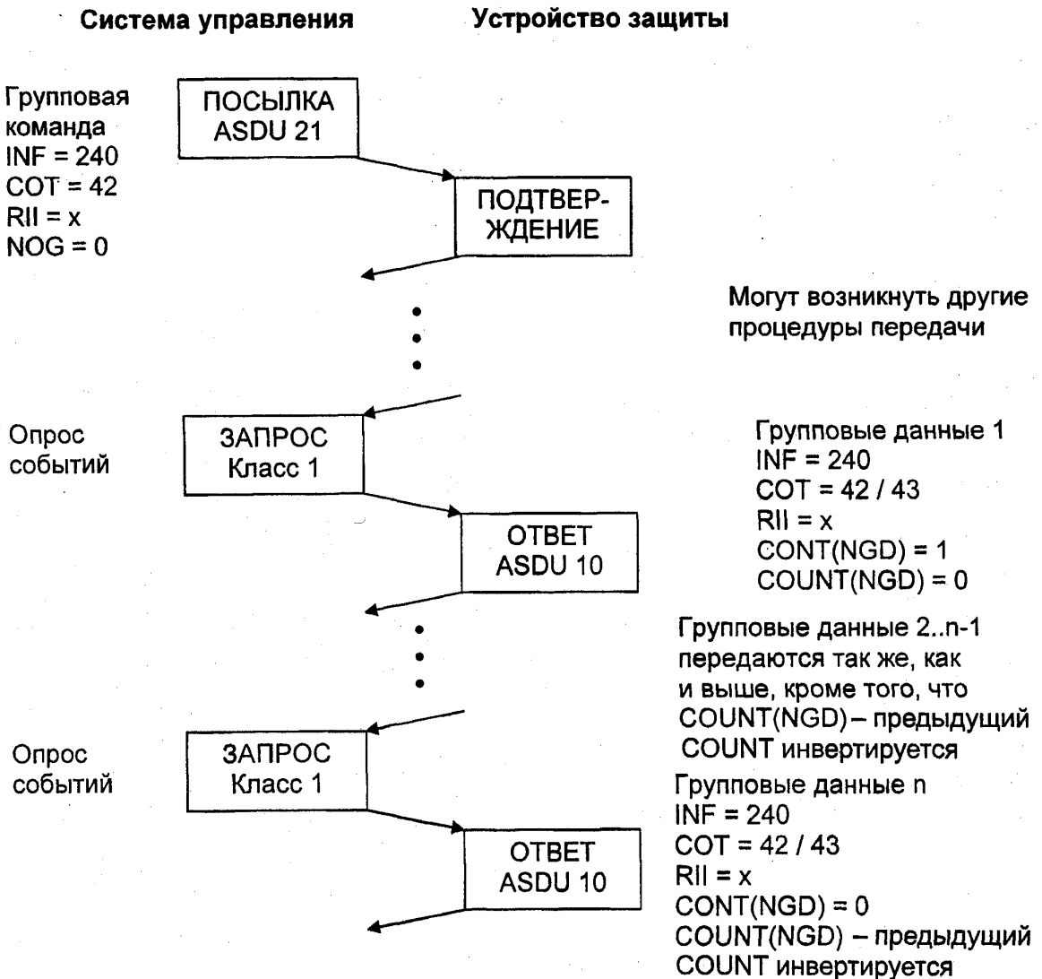
Рисунок 13 — Чтение заголовков всех определенных групп
