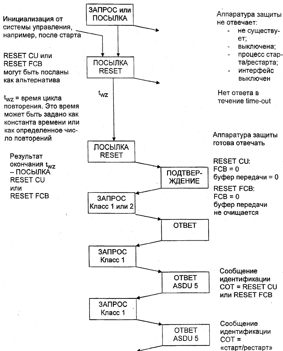
Рисунок 3 — Основная процедура инициализации
