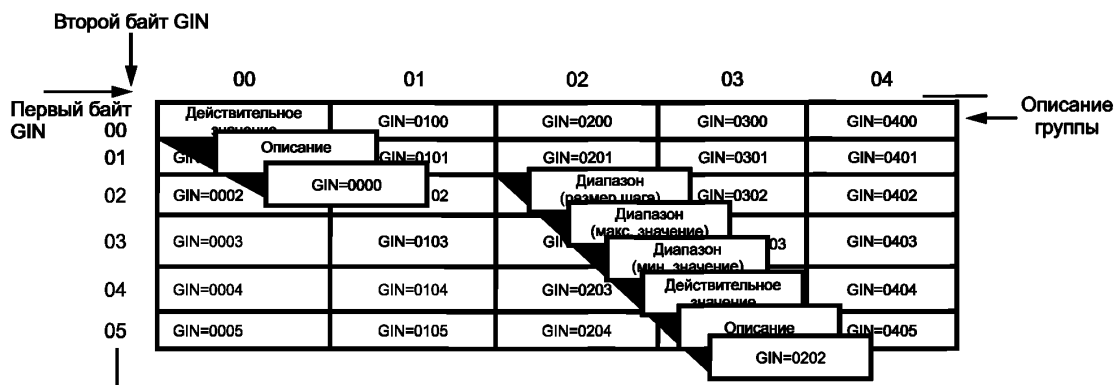
Рисунок 11 — Пример структуры директории
