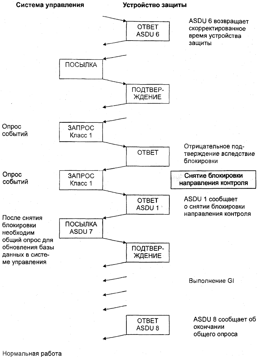
Рисунок 9 — Блокировка направления контроля (лист 2)
