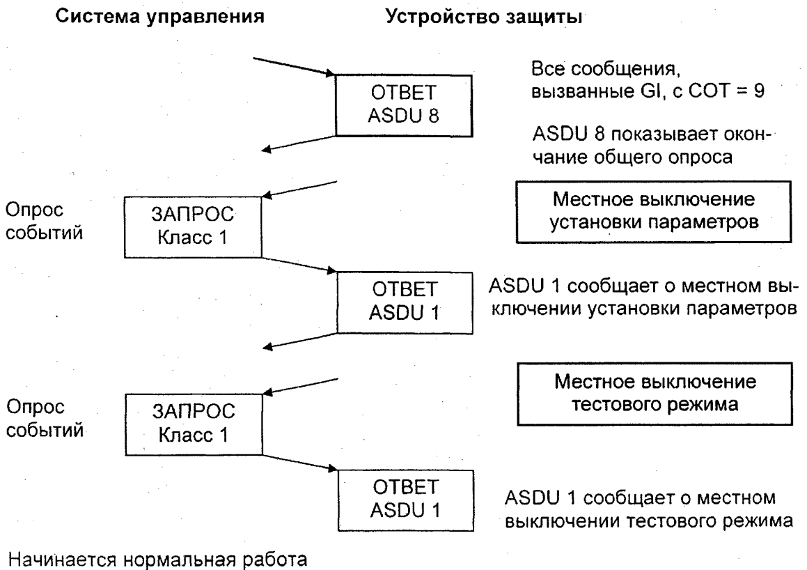
Рисунок 8 — Тестовый режим (лист 2)
