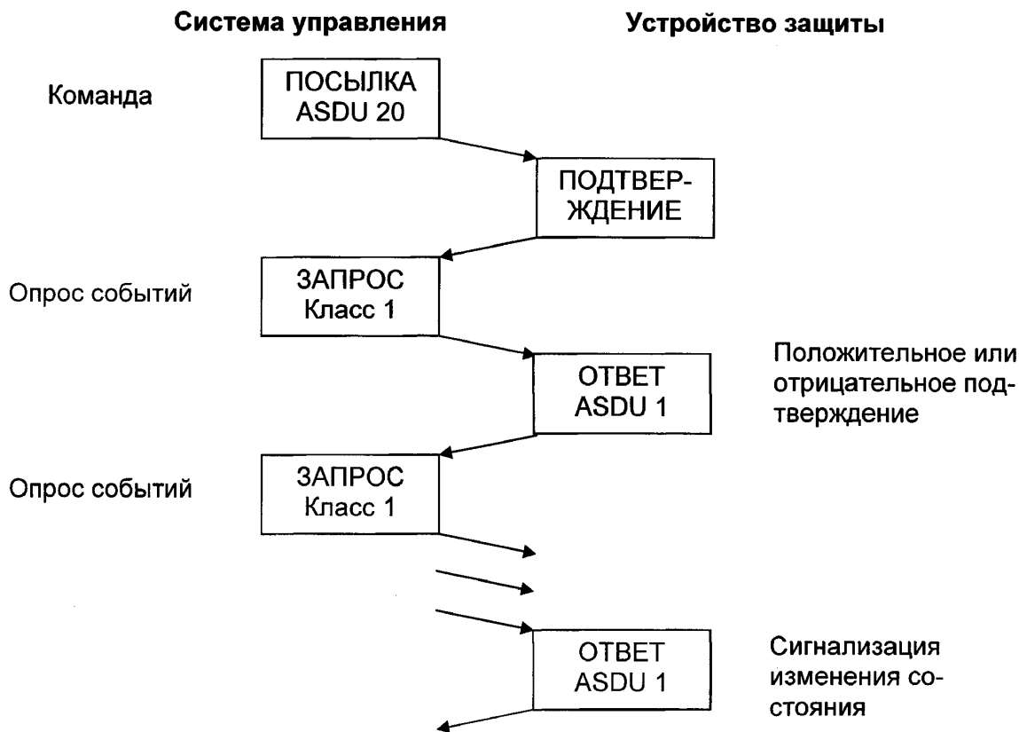
Рисунок 7 — Передача команд
