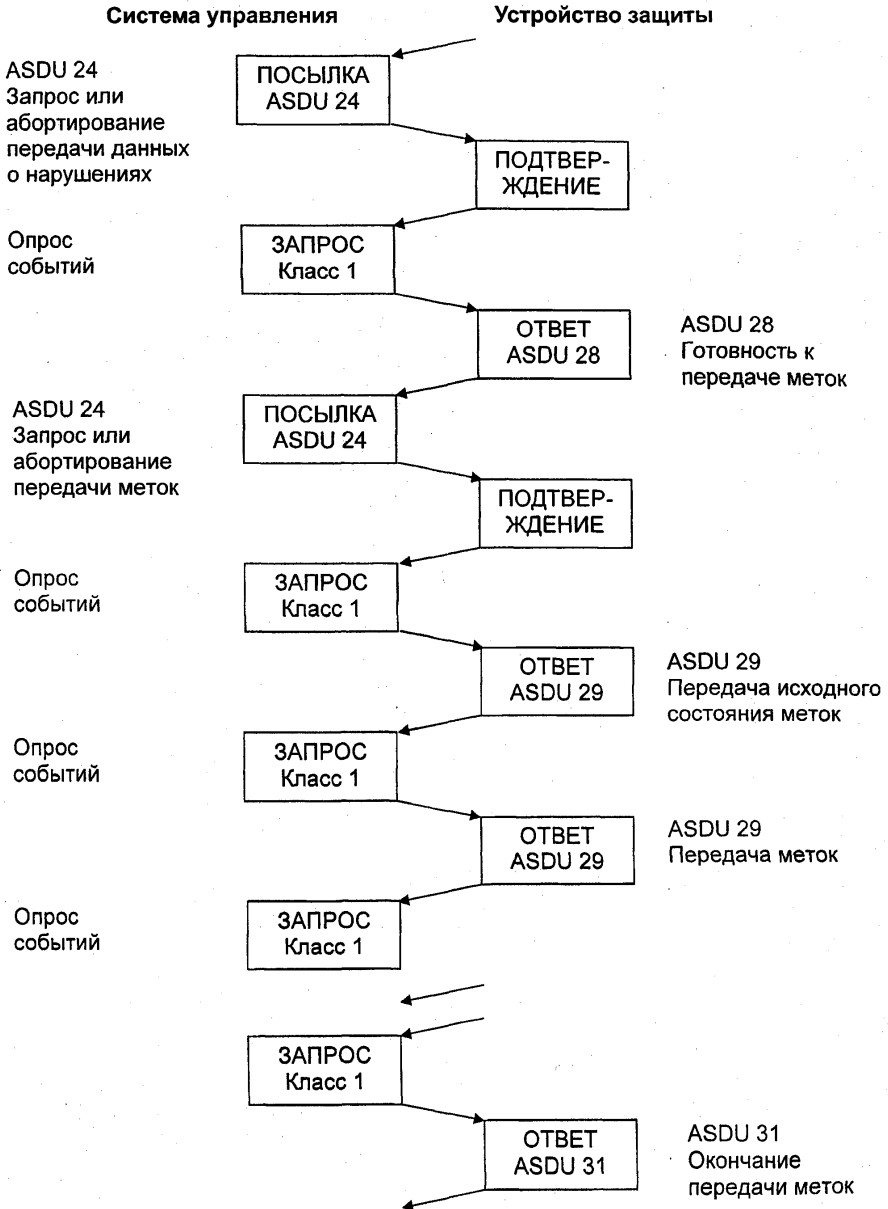
Рисунок 10 — Передача данных о нарушениях (лист 2)
