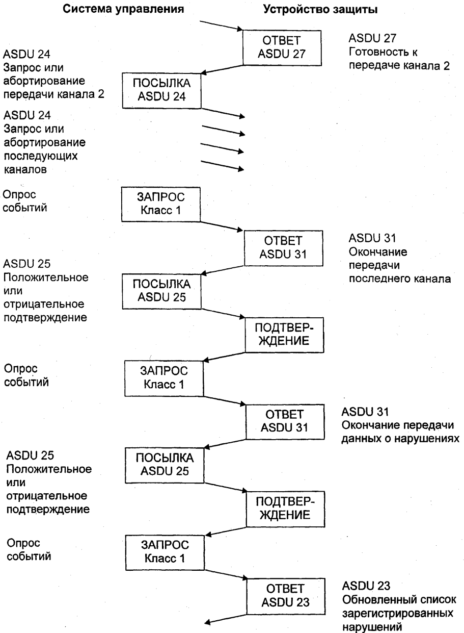
Рисунок 10 — Передача данных о нарушениях (лист 4)
