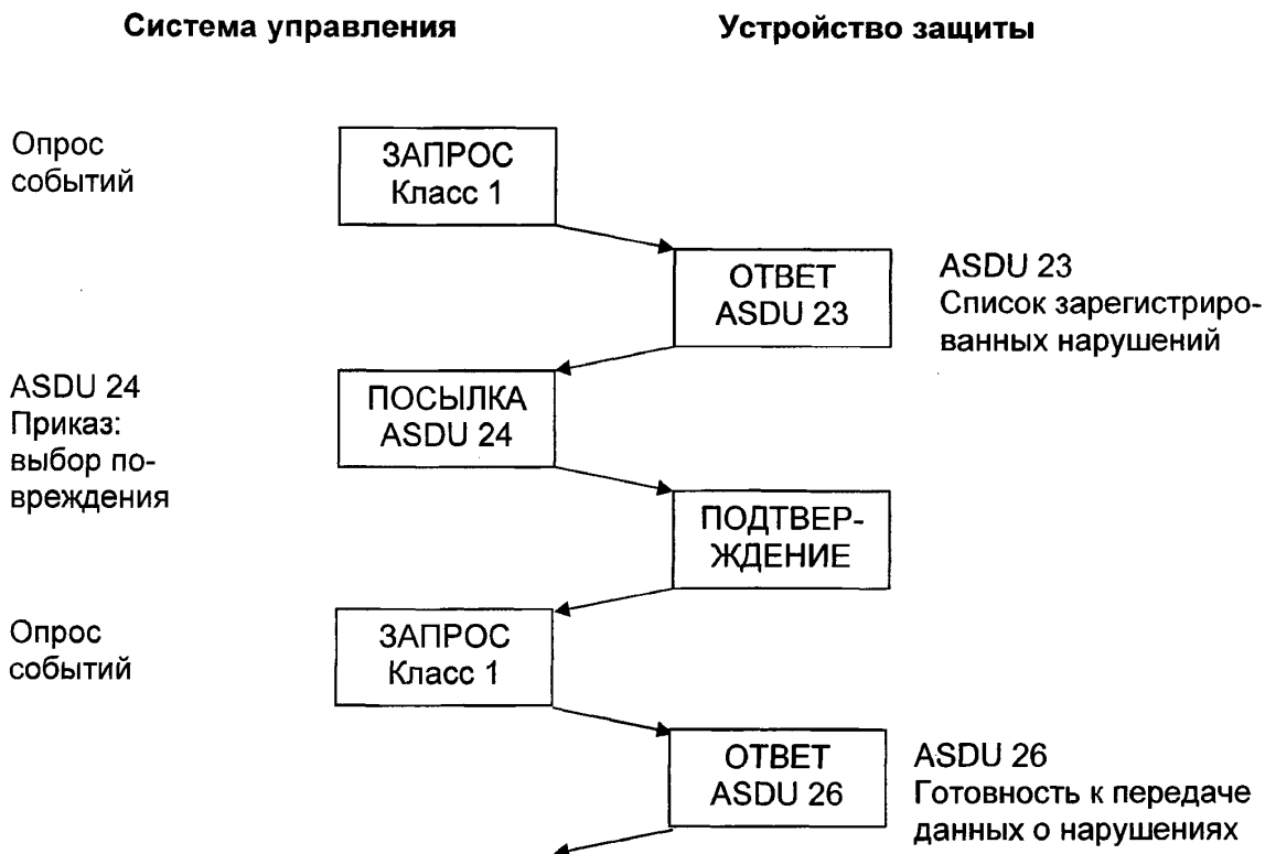
Рисунок 10 — Передача данных о нарушениях (лист 1)
