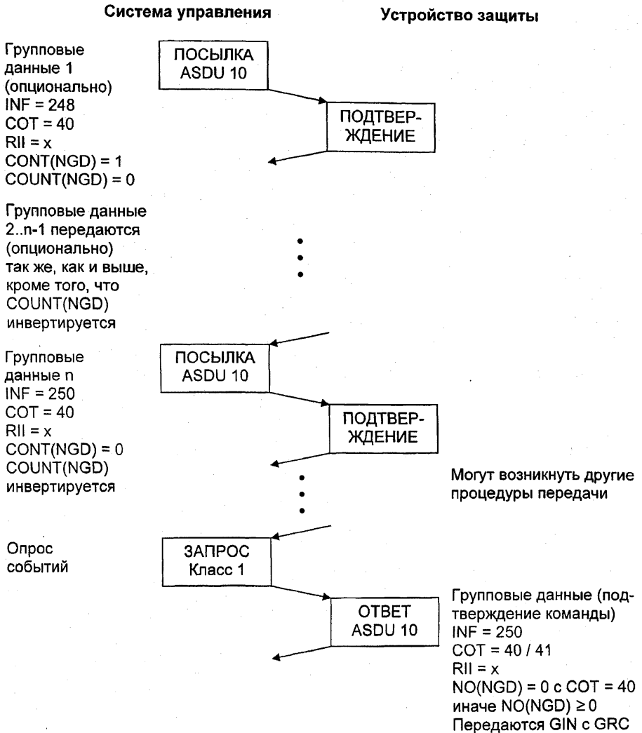
Рисунок 17 — Запись значений одиночных элементов
