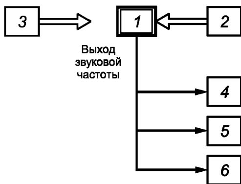
1 — испытуемое оборудование станции радиоконтроля; 2 — генератор 1; 3 — генератор 2; 4 — эквивалент нагрузки; 5 — вольтметр; 6 — измеритель нелинейных искажений
