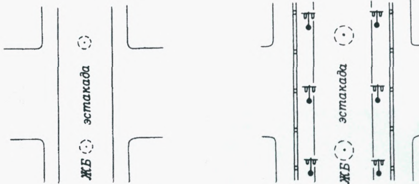
Эстакады-путепроводы
