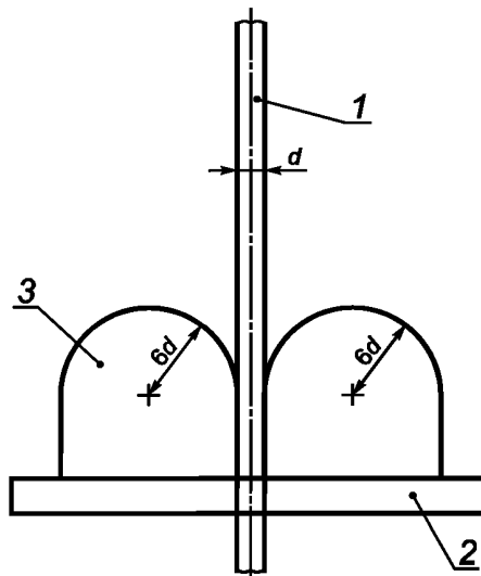
1 — образец сетевого электронагревателя; 2 — стальное основание; 3 — металлическая оправка; d — диаметр сетевого электронагревателя или первичная плоскость изгиба, если изготовитель не указал иное
