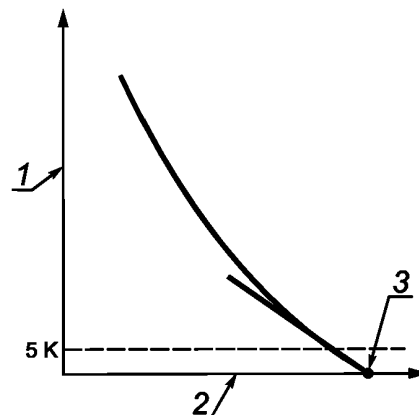
1 — температура образца минус температура воздуха в печи ( T_s - T_o ), К; 2 — температура в печи T_o , °С; 3 — зарегистрированное значение температуры T_s , °С
