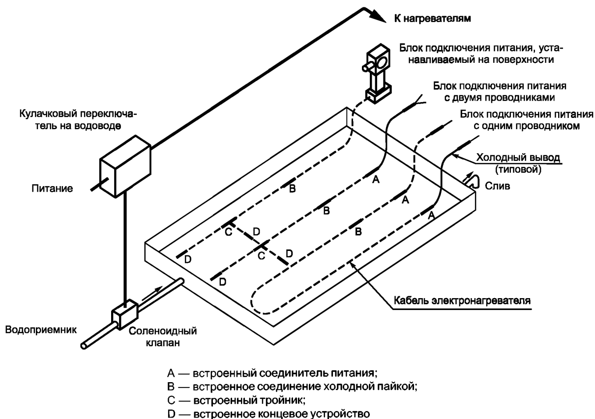
Рисунок 4 — Испытание встроенных компонентов на влагоустойчивость
