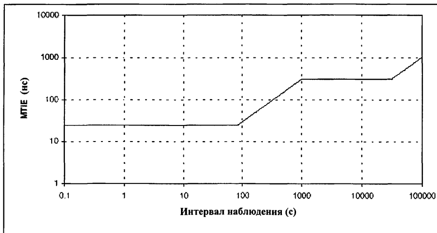
Рисунок 3/ETS 300 462-3: Сетевой допустимый предел для дрейфа фазы на выходах PRC, выраженный в МТИЕ
