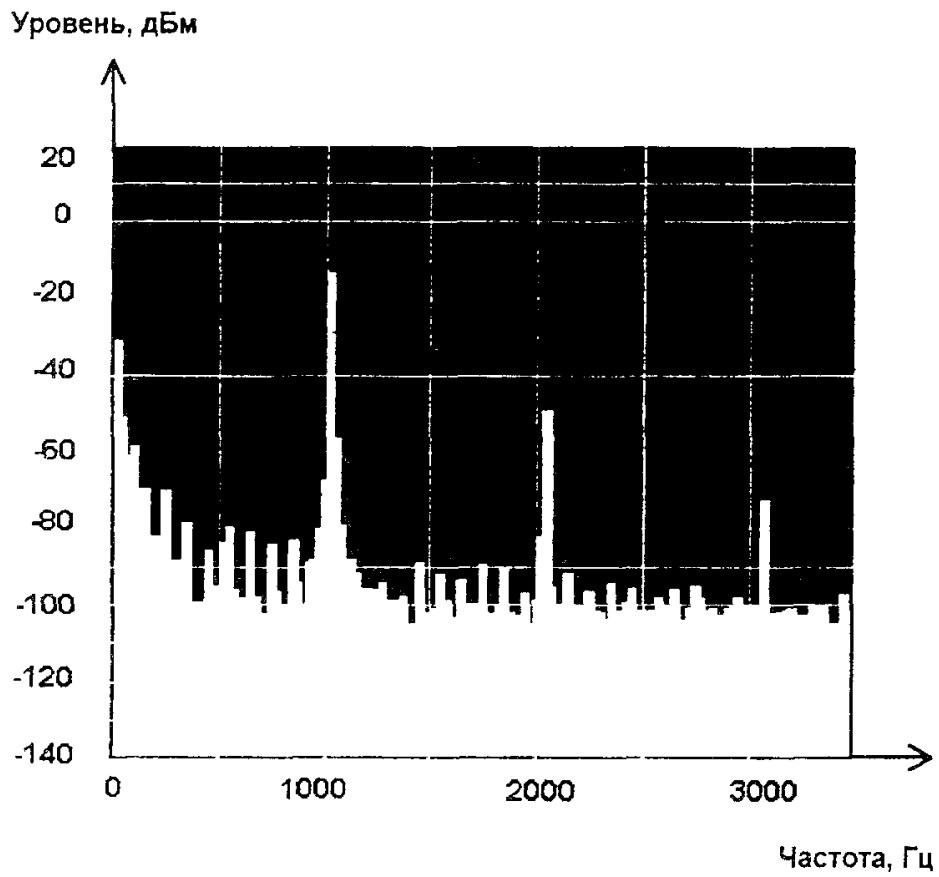
Рисунок 10 - Спектральная характеристика сигнала частотой 1020 Гц при наличии нелинейных искажений
