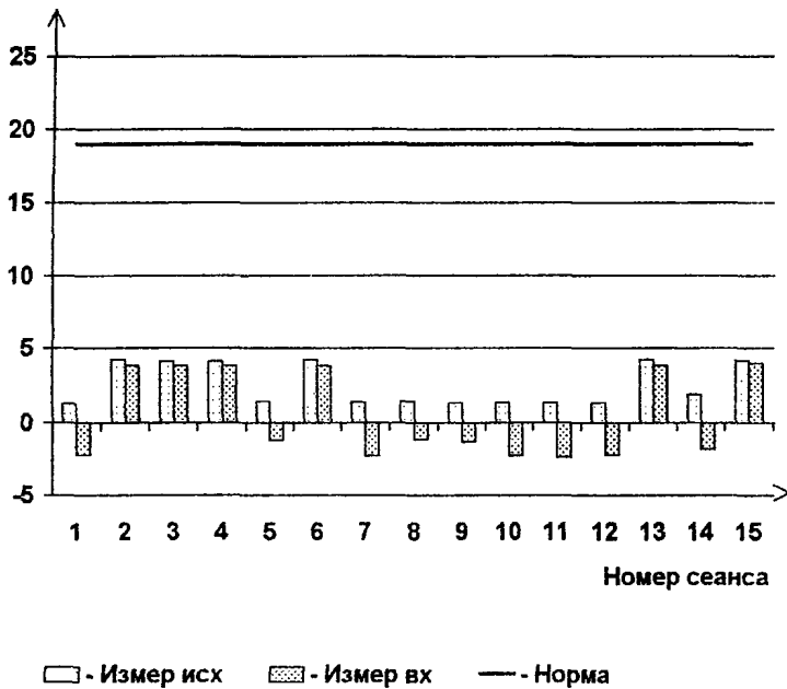
Рисунок 2 - Затухание сигнала на частоте 2400 Гц при анизотропности телефонных каналов
