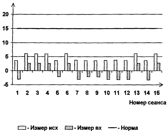
Рисунок 1 - Затухание сигнала на частоте 1020 Гц при анизотропности телефонных каналов
