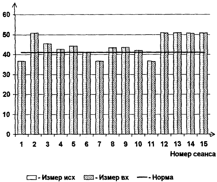
Рисунок 4 - Затухание сигнала на частоте 2400 Гц в каждом из 15 сеансов
