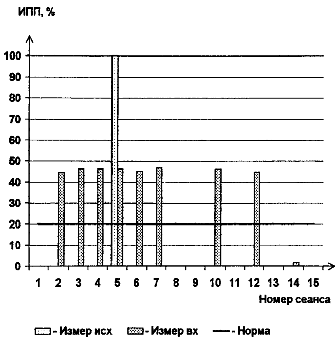
Рисунок 11 - Импульсные помехи и перерывы
