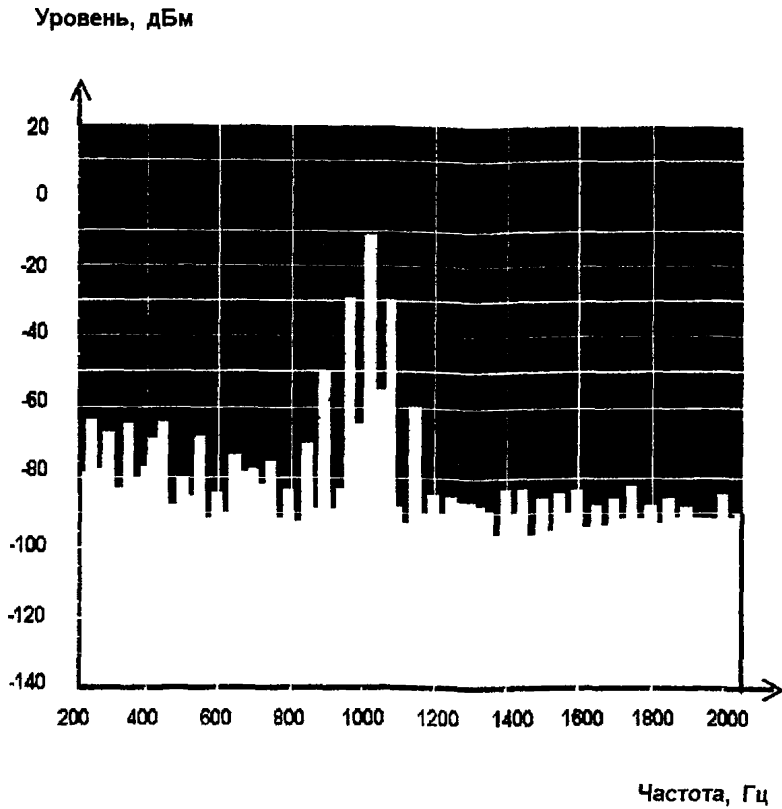
Рисунок 9 - Спектральная характеристика сигнала частотой 1020 Гц при наличии паразитной модуляции сигнала помехами источника питания
