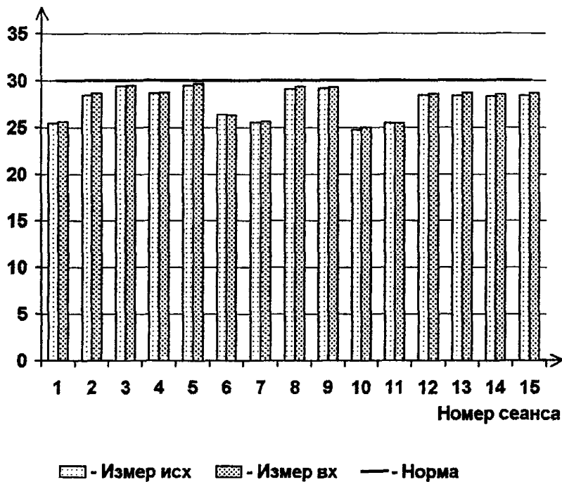
Рисунок 6 - Затухание сигнала на частоте 1020 Гц в каждом из 15 сеансов
