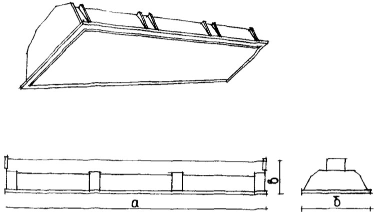
СВЕТИЛЬНИК ОВА-2x40
