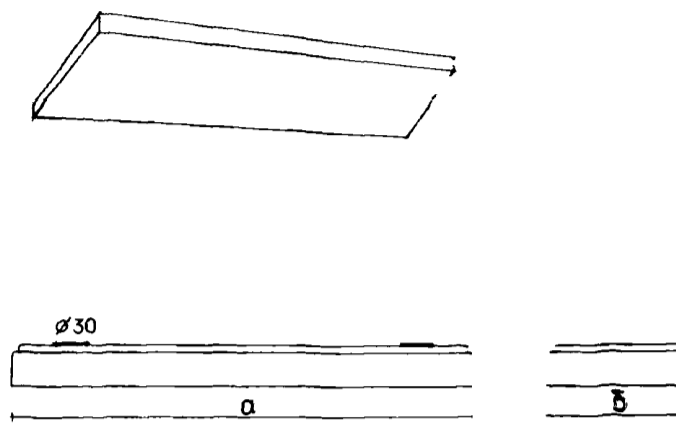
СВЕТИЛЬНИК ПЛ2А-2x40
