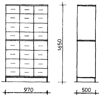
21 ШКАФ КАРТОТЕЧНЫЙ
