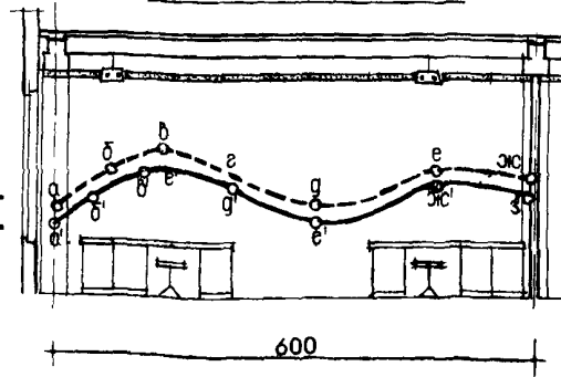
РАЗРЕЗЫ 2-2 и 2'-2'
