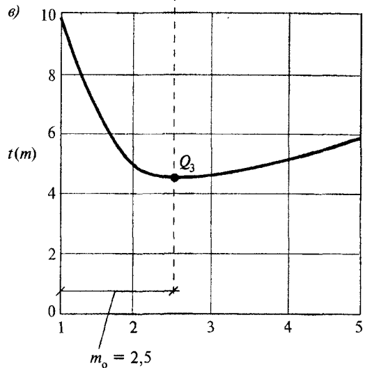
Рисунок 1. Зависимость расчетных экономических характеристик от повышения уровня теплозащиты в m раз ограждающих конструкций
