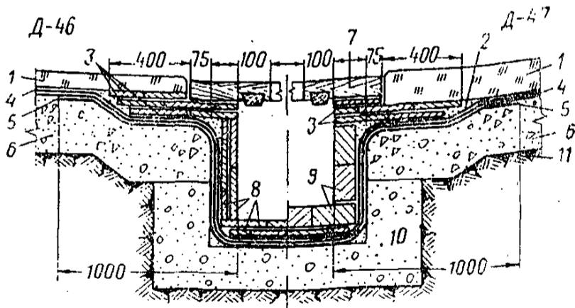
Рис. 9. Каналы в полах для стока воды, содержащей кислоты и щелочи
