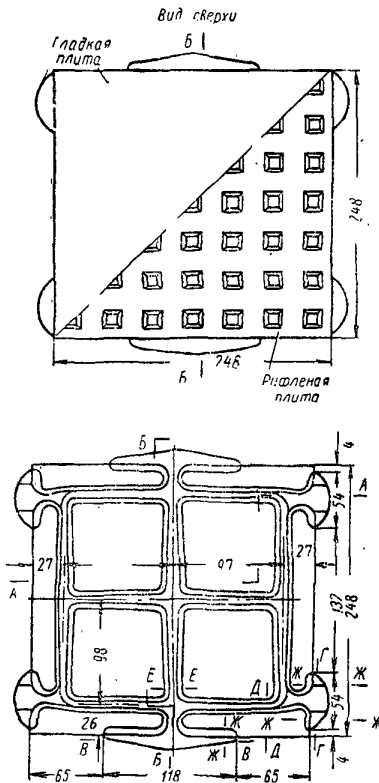
Рис. 7. Плита чугунная с опорными выступами для полов, укладываемая на песке. Общий вид. Вес плиты: гладкой 6,9 кг, рифленной 7,1 кг
