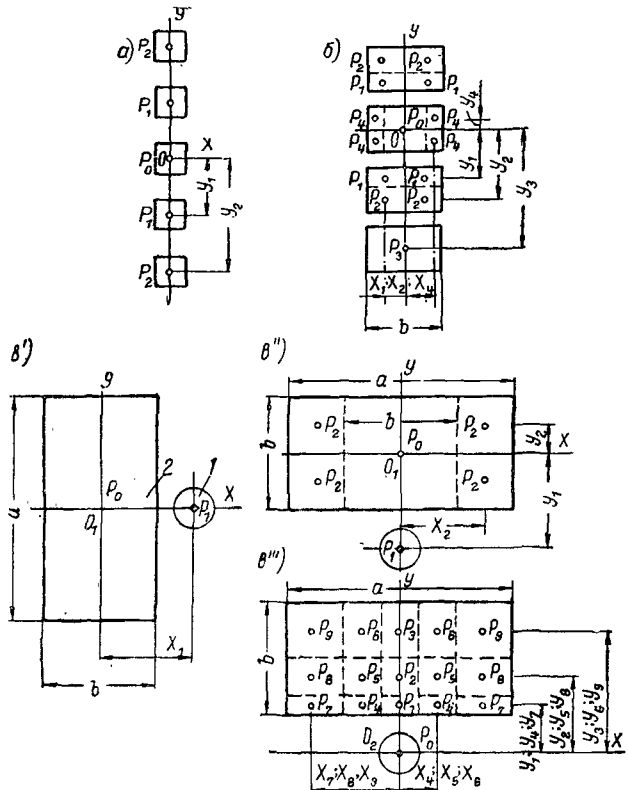
Рис. 4. Схемы расположения в плане нагрузок сложного вида, расчетного центра O , осей координат и разделенных следов нагрузок на элементарные площадки
