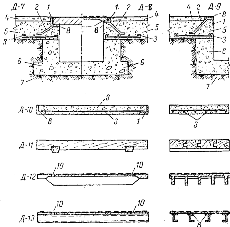
Рис. 2. Примыкание полов к каналам и приямам при отсутствии воздействия на пол жидкостей
