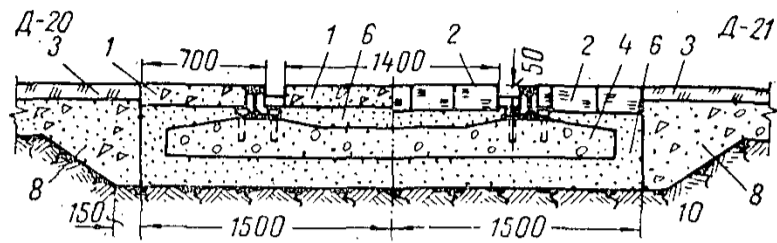
Рис. 4. Полы в зоне железнодорожных путей
