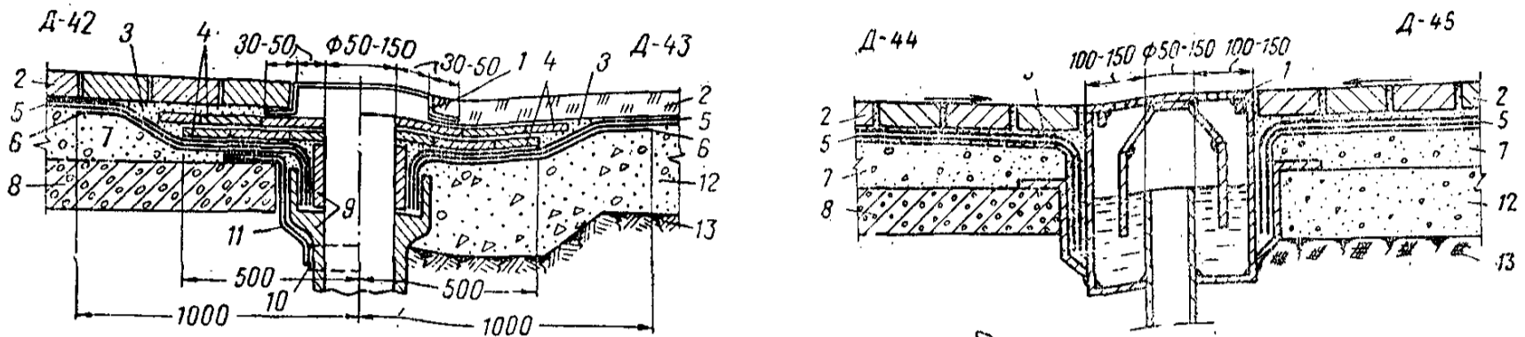
Рис. 8. Трапы в полах для стока воды, содержащей кислоты и щелочи
