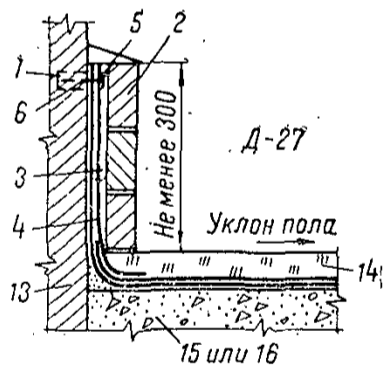
Рис. 5. Плинтусы при воздействии на пол жидкостей
