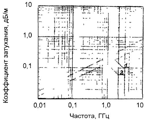
Рис.43. Частотная зависимость коэффициента затухания 1 – РК-50-7-58, Г, 2 - РК 50-7-59, Г
