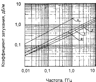
Рис 60 Частотная зависимость коэффициента затухания 1 - РД 50-1-11, 2 - РД 75-3-11, РД 75-3-12; 3 - РД 75-1-11, 4 - РД 100-0,6-22
