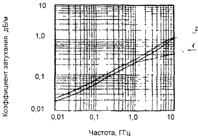
Рис 37 Частотная зависимость коэффициента затухания 1 - РК 75-7-15, 2 - РК 100-7-11
