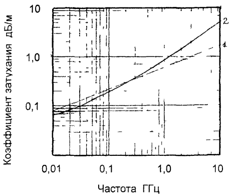
Рис 15 Частотная зависимость коэффициента затухания 1- РКОГ-2М 2- РК 50-1,5-31
