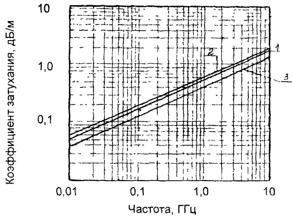
Рис.24. Частотная зависимость коэффицента затухания 1- РК 75-2-21, 2- РК 75-2-22, 3- РК 50-3-21 и РК 75-3-21
