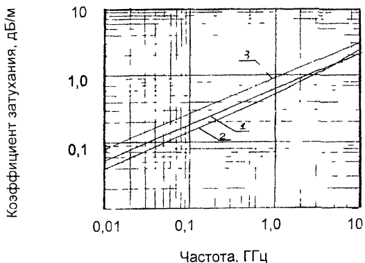
Рис 12 Частотная зависимость коэффициента затухания 1 – РК 50-2-11, 2 – РК 50-3-11 и РК 50-3-13, 3 – РК 50-1,5-11
