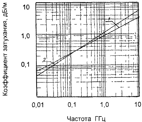
Рис 19 Частотная зависимость коэффициента затухания 1 - РК 75-1,5-22 2 - РК0ГТ
