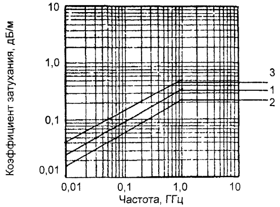
Рис. 71 Частотная зависимость коэффициента затухания 1 – РИ 75-4-11, 2 – РИ 75-7-11; 3 – РИ 75-4-12
