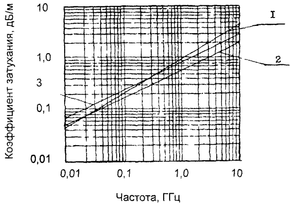
Рис.23. Частотная зависимость коэффицента затухания 1- РК 50-2-24; 2- РК 50-2-25,Т,28,29; 3- РК 50-2-26
