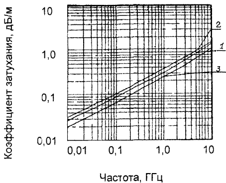
Рис 35 Частотная зависимость коэффициента затухания 1 - РК 75-4-15, 2 - РК 75-4-16, 3 - РК 50-7-11
