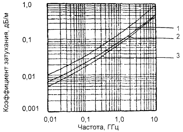
Рис. 76. Частотная зависимость коэффициента затухания 1 – РК 75-13-11, 2 – РК 75-13-32, 3 – РК 75-17-31
