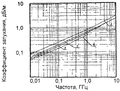
Рис 13 Частотная зависимость коэффициента затухания 1- РК 75-1,5-11, 2- РК 75-2-12, 3- РК 75-2-11, 4 – РК 75-3-16AY
