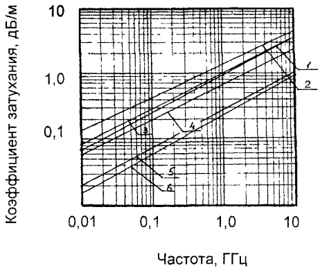
Рис 65. Частотная зависимость коэффициента затухания 1 - РК 50-1-23С; 2 - РК 50-1-25С, 3 - РК 50-1,5-23С, 4 - РК 50-2-27С, 5 - РК 50-4-31С; 6 - РК 50-4-32С
