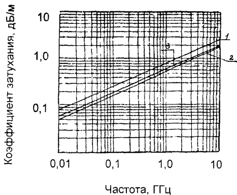
Рис 21 Частотная зависимость коэффициента затухания 1- РК 50-1,5-21 и РК 75-1,5-21; 2- РК 50-2-21; 3- РК 50-2-22
