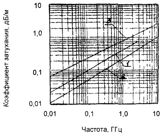
Рис 36 Частотная зависимость коэффициента затухания 1 - РК 75-9-18, 2 - РК 75-9-14 3 - РК 75-7-18
