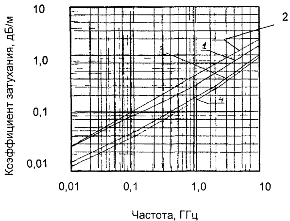
Рис 28 Частотная зависимость коэффициента затухания 1- РК 75-4-115 и РК 50-4-11, 2- РК 50-4-14 ОП, 3 РК 50-9-12 4- РК 50-11-11
