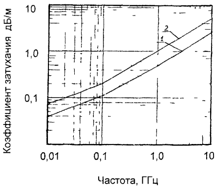
Рис 16 Частотная зависимость коэффициента затухания 1- РК 75-3-34 2- РК 75-1,5-32
