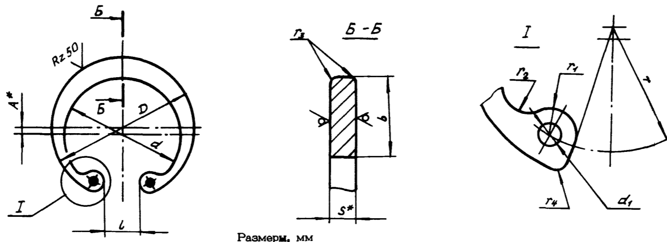
Размеры, мм
