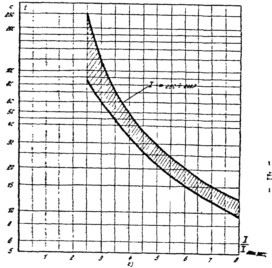
Рис. II. Время-токовая характеристика срабатывания выключателей: а - АЗ110; б - АЗ120; в - АЗ130; г - АЗ140
