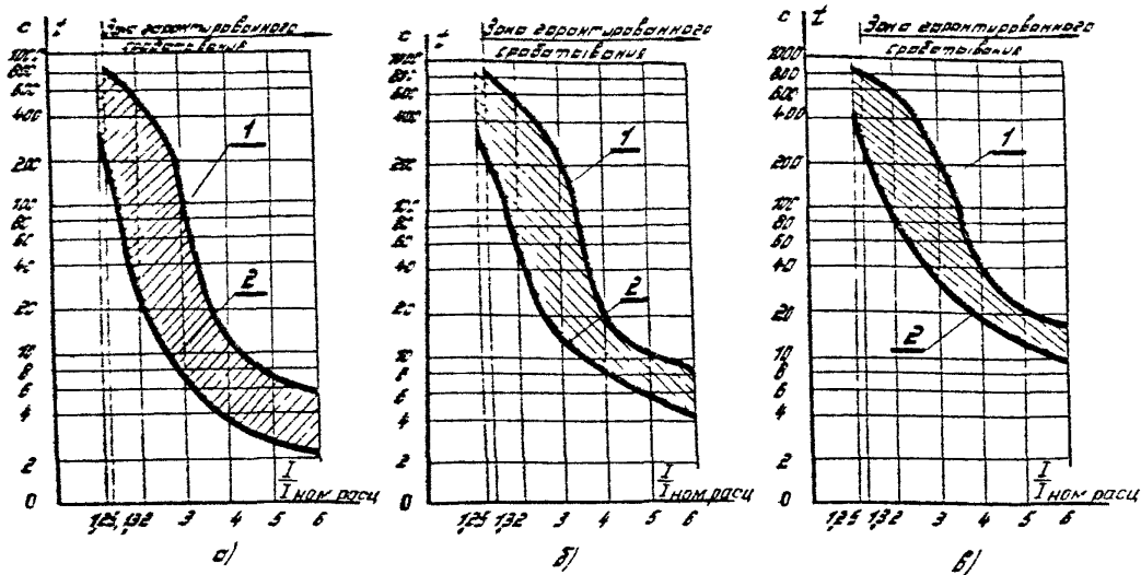
Рис.10. Защитные характеристики полупроводникового распределителя постоянного тока при уставке времени срабатывания: а - 4 с; б - 8 с; в - 16 с.
