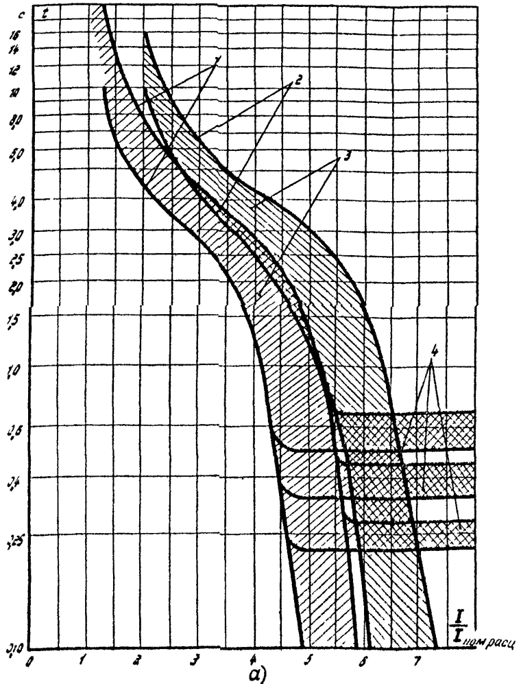
Рис.6. Защитные характеристики выключателей: а) АЕМ 10Н и АЕМ 15С, АЕМ 20Н и АЕМ 20С с номинальным током срабатывания МТЗ 1500 А; б) АЕМ 20Н и АЕМ 20С с номинальным током срабатывания МТЗ 1800 А I — при минимальных уставках на шкалах замедленного и мгновенного срабатывания электромагнитного максимального расцепителя тока;
