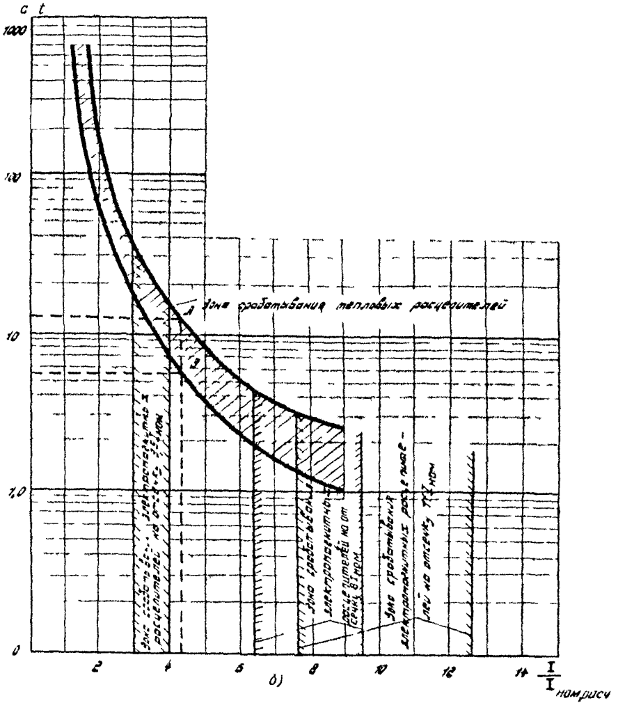
Рис.14. Время-токовые характеристики выключателя серии АП-50 на номинальный ток: а - 10 А; б - 16 А
