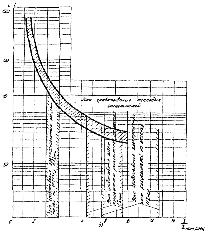
Рис.13. Время-токовые характеристики выключателя серии АД-50 на номинальный ток: а - 4 А; б - 6,4 А
