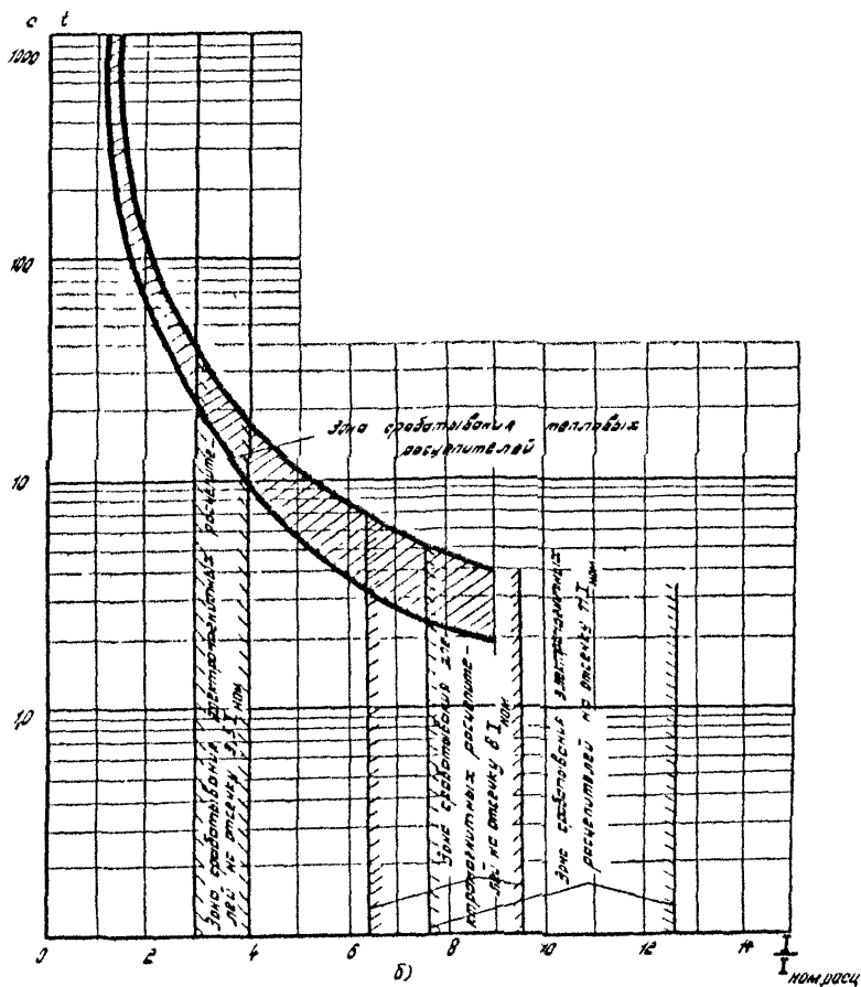
Фиг.15. Время-токовые характеристики выключателя серии АП-50 на номинальный ток:
