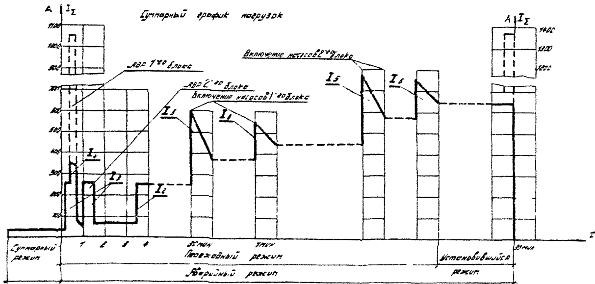
Рис.2. График нагрузок аварийного почасового режима для ТЭС с блоками мощностью 150-200 МВт П р и м е ч а н и е. Время включения насосов уплотнения (30 с) и смазки (1 мин) принято условно. В общем случае моменты включения указанных насосов для 1-го и 2-го блоков не совпадают, что учтено в суммарном графике нагрузок
