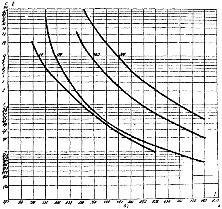
Рис.16. Время-токовые характеристики предохранителей ПР-2: \alpha - I_{\text{ном.пл.вст}} = 60+200 \text{ A} ; \beta - I_{\text{ном. пл.вст}} = 15+15 \text{ A}
