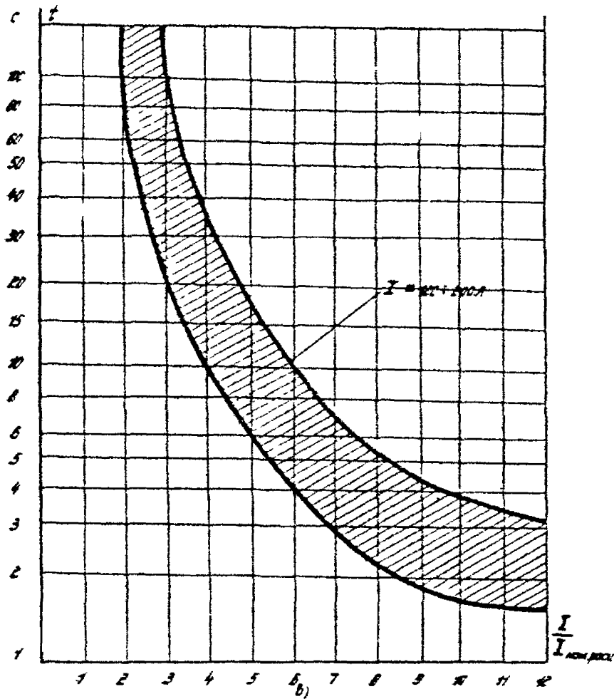
Рис. II. Время-токовая характеристика срабатывания выключателей: а - АЗ110; б - АЗ120; в - АЗ130; г - АЗ140
