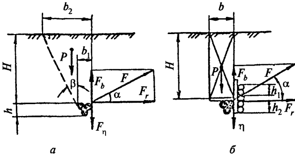
а — якорь без щита; б — якорь со щитом
