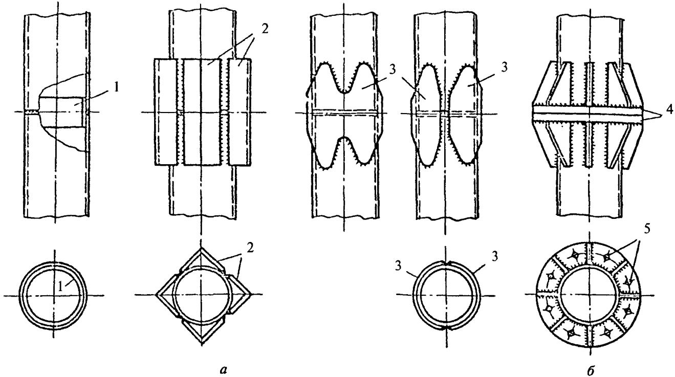
а — сварных; б — болтовых; 1 — подкладка, 2 — уголовые накладки, 3 — фигурные накладки, 4 — фланцы, 5 — болты
