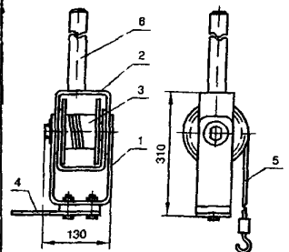
ЛЕБЕДКА РУЧНАЯ РЫЧАЖНАЯ 0,65т
