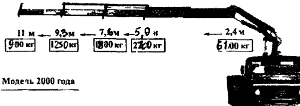
Кран-манипулятор - БАКМ-1600
