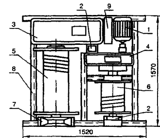
ЛЕБЕДКА ЭЛЕКТРИЧЕСКАЯ 5т (двухбарабанная)
