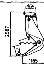
ИГ-811
