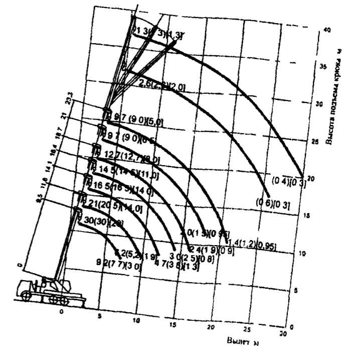
Грузовысотные характеристики Полный опорный контур Зоны работы +45° (±125°) [360°]
