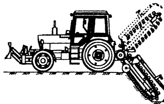
Рис.5 ЭТЦ-1609
