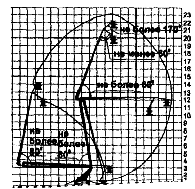
Зона обслуживания МШТС-23
