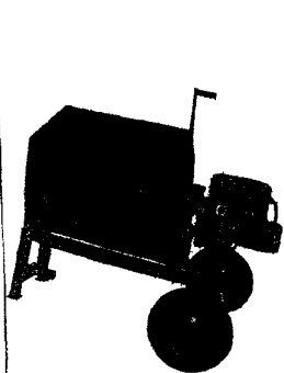
Рис. 1 Растворосмеситель С0-46В
