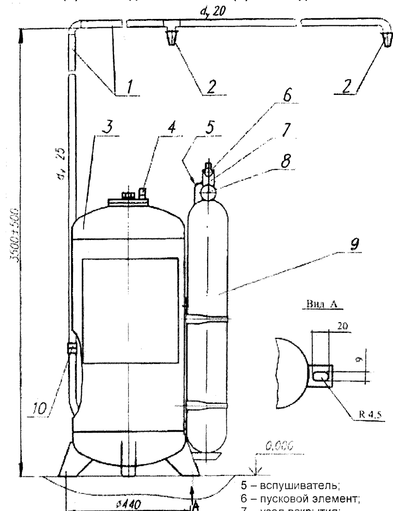
Общий вид модуля «Лавина» МПП(Н)-100-07-КД-2-БСГ-У2 и МПП(Н)-100-08-КД-2-БСГ-У2
