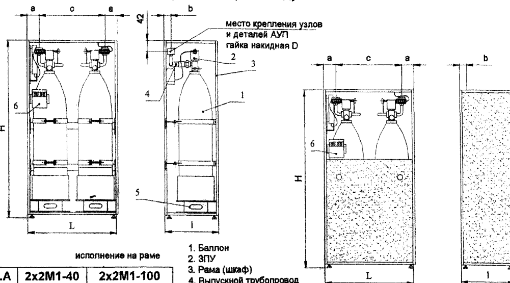
Габаритный чертеж модуля 2М1.
