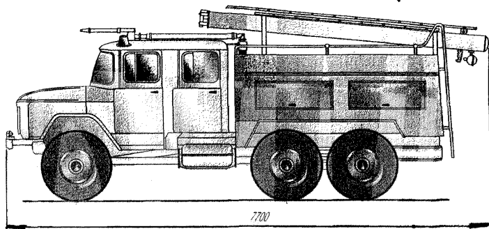
Рис.1 АЦ-2,5-40(ЗИП-131)-6ВР
