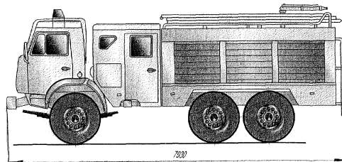
Рис.4 АЦ-4,0-40(Упан-5557)-9Б
