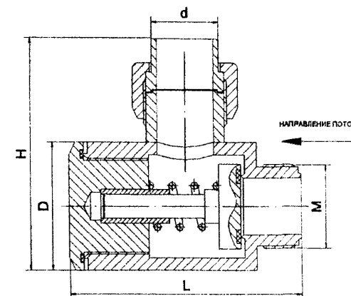
КЛАПАН ОБРАТНЫЙ УГЛОВОЙ
