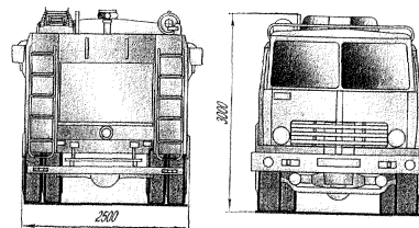
Рис. 8 АЦ-7,0-40(КамАЗ-532150)-21БР
