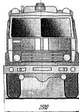
Рис.6 АЦ-5,0-40(КамАЗ-43114)-20БР
