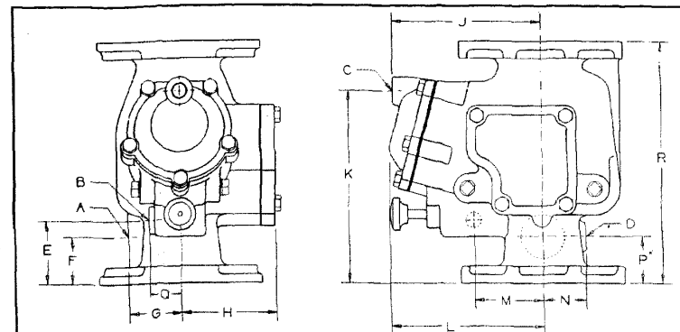
4" (100 мм) Клапан
