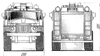
Рис. 7 АЦ-6,0-40(Урал-5557)-12БР
