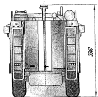
Рис.6 АЦ-5,0-40(КамАЗ-43114)-20БР
