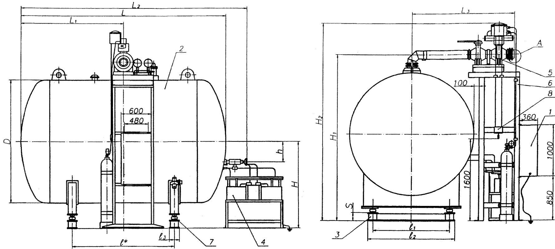
1 – Шкаф управления; 2 – Резервуар РЖУ; 3 – Опора резервуара; 4 – Агрегат холодильный (ХА); 5 – Запорно-пусковое устройство (ЗПУ); 6 – Опора ЗПУ; 7 – Тензорезисторные датчики силы; 8 – Устройство местного пуска
