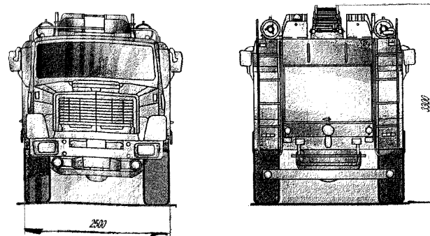
Рис.3 АЦ-3,0-40(ЗИП-4334)-3ВР
