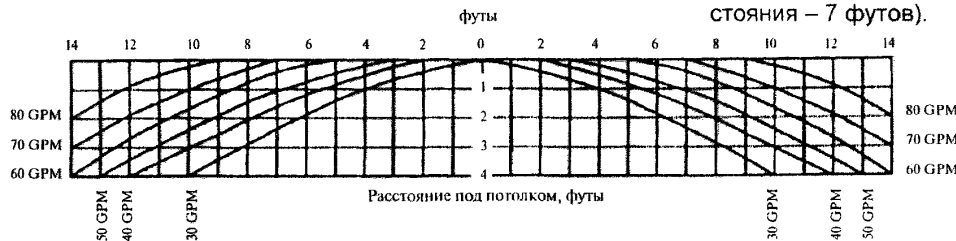
Рисунок D Карты номинального орошения для спринклеров модели F895 Ду 5/8" и 3/4" с плоской и вогнутой розеткой увеличенной площади орошения
