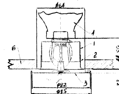
Схема монтажа оросителя скрытого декоративной крышкой
