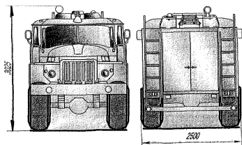
Рис.4 АЦ-4,0-40(Упан-5557)-9Б
