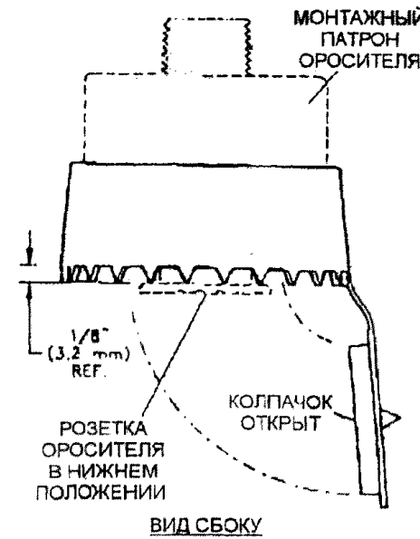
Рис.4 Защитный колпак
