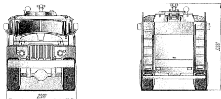
Рис. 9 АЦ-8,0-40(Урал-4320)-25БР
