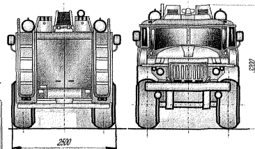
Рис.5 АЦ-5,0-40(Упан-5557)-11Б
