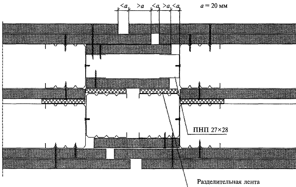
Рисунок 20 — Схема устройства деформационного шва в перегородке С 115.2
