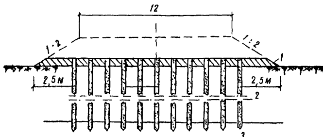
Рис.2. Поперечное сечение насыпи земляного полотна со сваями: 1-рабочая платформа; 2-иольдзевая глина; 3-моренный суглинок
