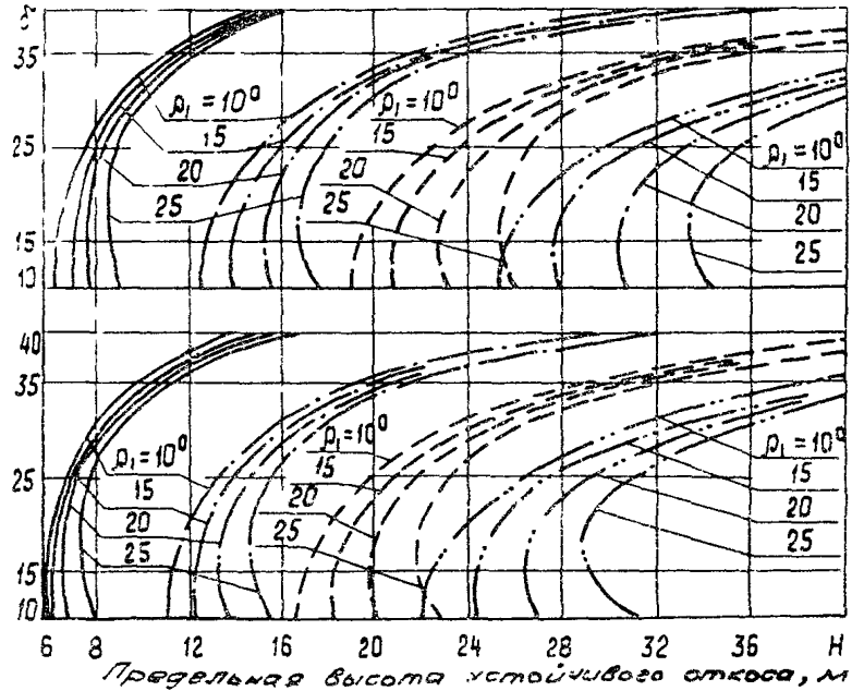
Рис. 7. Номограммы для определения предельной высоты устойчивого откоса при наличии двух или более систем поверхностей ослабления, падающих в сторону откоса под различными углами, одна из которых совпадает с откосом (для некоторых расчетных сочетаний) / расчетная схема У1/:
