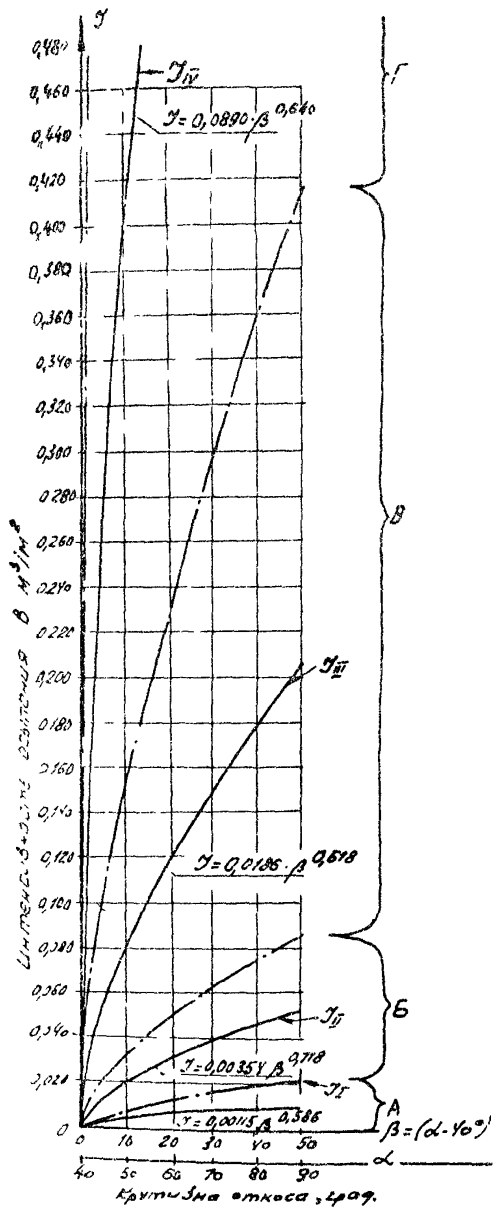
Рис. 3. Зависимости интенсивности осипания от крутизны откосов для различных по степени устойчивости групп пород: J_I, J_{II}, J_{III}, J_{IV}, J_V - средние значения интенсивности осипания пород соответствующих групп; — границы между группами
