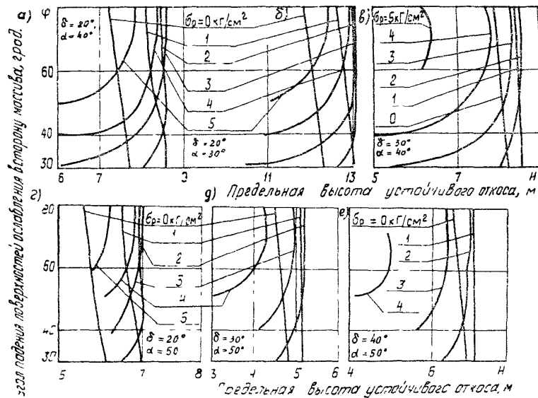
Рис. 10. Номограммы для определения предельной высоты устойчивого откоса с углом наклона \delta при наличии двух или более систем поверхностей ослабления, одна из которых имеет падение в сторону выемки под углом \alpha ( \alpha < \delta ), а другая - в сторону массива под углом \varphi (для некоторых расчетных сочетаний) / расчетная схема УШ/
