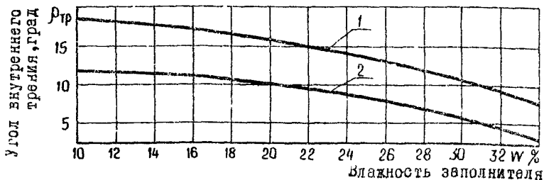
Рис. 10. Зависимость угла внутреннего трения по контактам поверхностей ослабления \beta_{тр} от влажности заполнителя:
