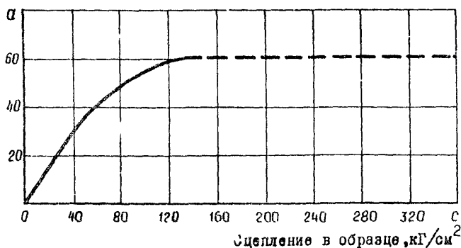
Рис. 12. Зависимость коэффициента \alpha от величины сцепления в образце (по данным ЦНИИСа)
