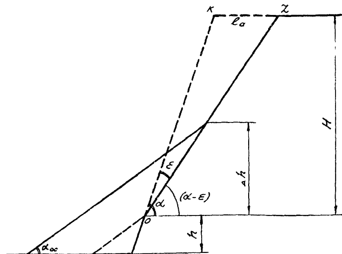
Рис.7. Схема к расчету уположения откоса во времени (за счет осыпания продуктов выветривания)
