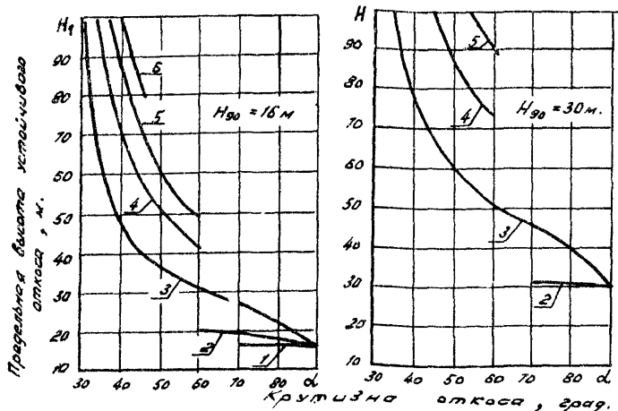
Рис. 6. Пределная высота устойчивого откоса при расчете по схеме X (для некоторых частных случаев):
