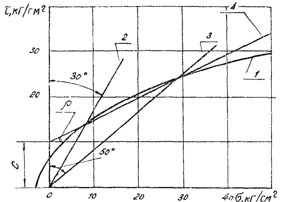
Рис. 8. Пример построения для получения значений \sigma и \rho в образце:
