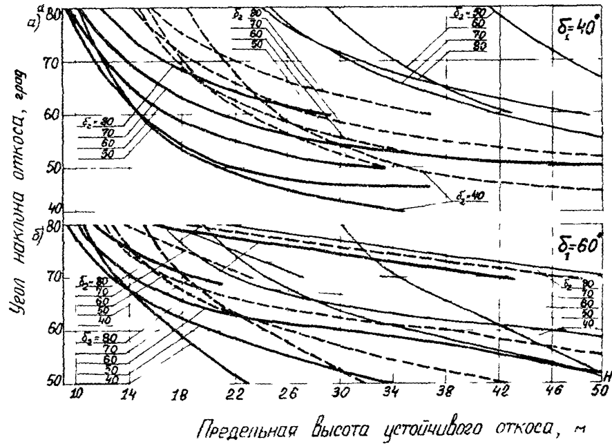
Рис. II. Номограммы для определения предельной высоты устойчивого откоса, при расчетной схеме, учитывающей объемное расположение поверхностей ослабления (для некоторых расчетных сочетаний) / расчетная схема XI/:
