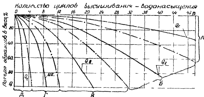
Рис. 1. Зависимости потерь образцов в весе (за счет фракций менее 10 мм) от количества циклов высушивания — водонасыщения для различных по степени устойчивости групп пород: Q_1, Q_{II}, Q_{III}, Q_{IV}, Q_V — средние значения потерь в весе пород соответствующих групп; — — — — — границы между группами
