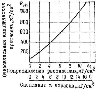
Рис. 9 Корреляционная зависимость R_{отн} от \sigma (по данным ЦНИИСа)
