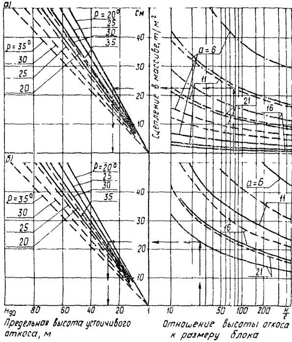
Рис.1. Номограммы для определения предельной высоты устойчивого вертикального откоса при благоприятном расположении поверхностей ослабления (расчетная схема I): а — — — — C = 100\text{Т/м}^2 ; - - - - C = 600\text{Т/м}^2 ; - - - - C = 1100\text{Т/м}^2 ; б — — — — C = 1600\text{Т/м}^2 ; - - - - C = 2100\text{Т/м}^2 ; - - - - \gamma_{об} = 2,5\text{Т/м}^3 ; - - - - \gamma_{об} = 2,0\text{Т/м}^3
