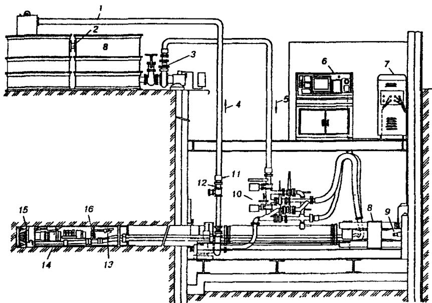
Рис. 5.10. Схема установки для прокладки коммуникаций способом микротоннелирования
