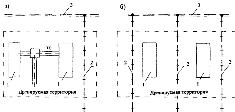
Рис. 6.1. Схемы дренажа: а) головного; б) систематического
