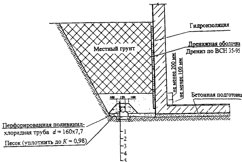
Рис. 6.3. Схема пристенного дренажа с применением поливинилхлоридных труб и дренажной оболочки «Дренаж» 1 – песок K_{\phi} > 5 м/сек; 2 – дорнит или минерально-волокнистый материал по ОСТ 33-10-73; 3 - гранитный щебень размером 3-10 мм; 4 - Бетон В15; 5 – гранитный щебень, втрамбованный в грунт
