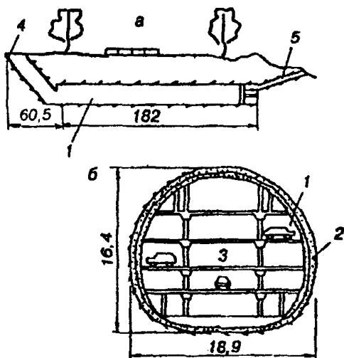
Рис. 5.3. Продольный разрез (а) и поперечный разрез (б) подземной автостоянки в г. Ландесберге (Германия) 1- стояночные места; 2- обделка; 3- проезд; 4- въезд-выезд; 5- аварийный выезд; (расстояние в метрах)
