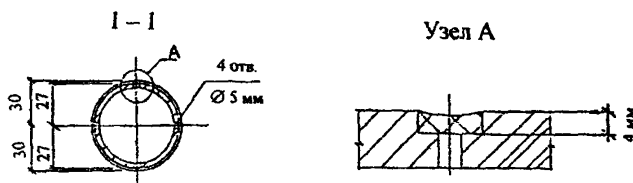
Рис. 7.1. Конструкция трубы-инъектора
