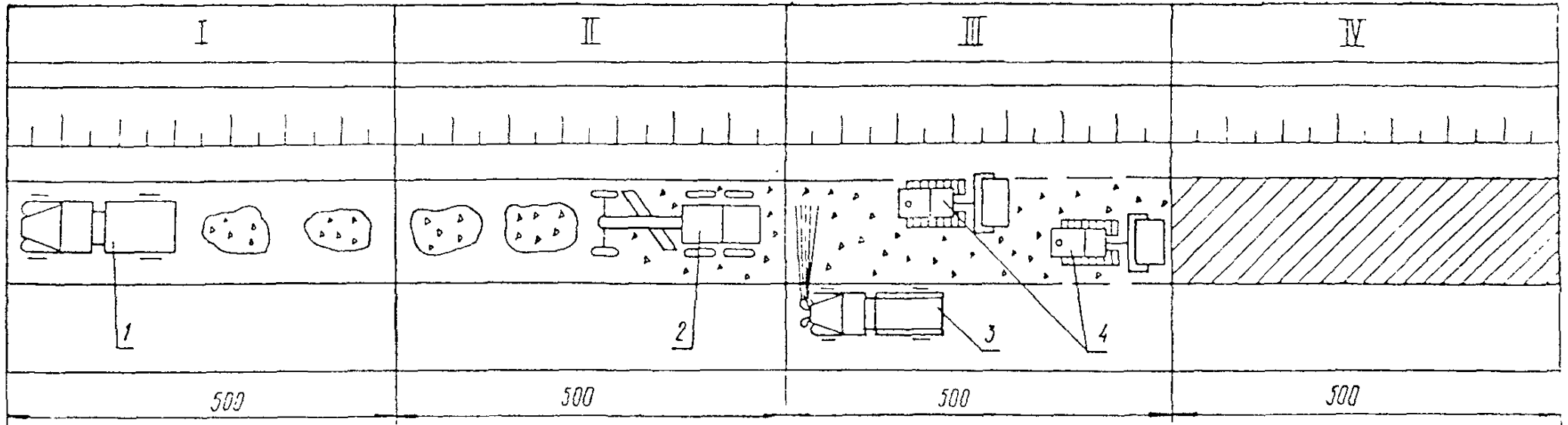
Рис. 1. Технологическая схема укрепления обочин щебнем:
