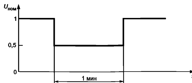
Рисунок В.3 — Провалы напряжения \Delta U = 50\%
