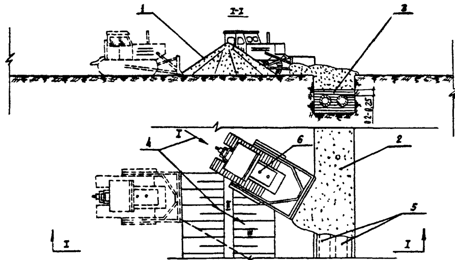
Рис.16. Засыпка теплосетей бульдозером. Схема организации работ: I, II, III - захватки засыпки грунта; I - отвал грунта; 2 - засыпанная траншея; 3 - грунт, засыпанный вручную и утрамбованный; 4 - направление движения бульдозера; 5 - трубы теплосети; 6 - бульдозер
