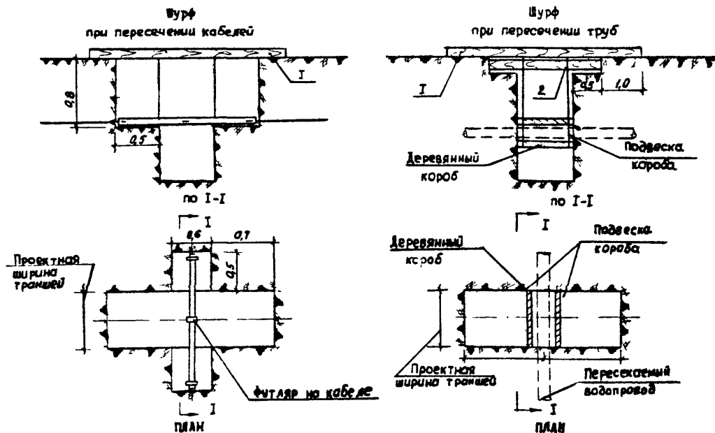
Рис.2. Организация работ:
