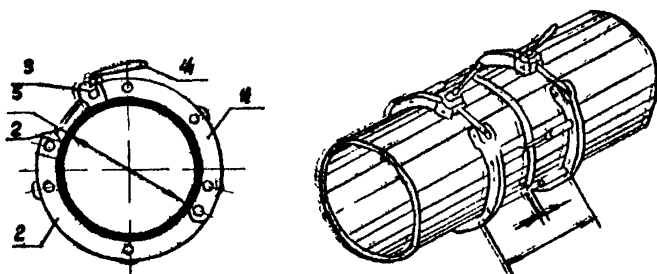
Рабочие чертежи винтового центриатора разработаны трестом "Мособлоргтехстрой", черт. 3-0-0-0.
