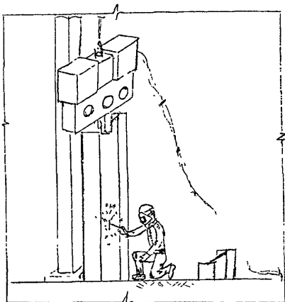
Рисунок 7 – Прорезание отверстия в шпунте
