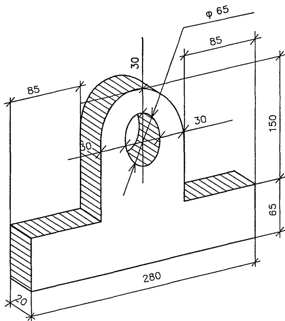
Рисунок 8 - Съемная монтажная петля
