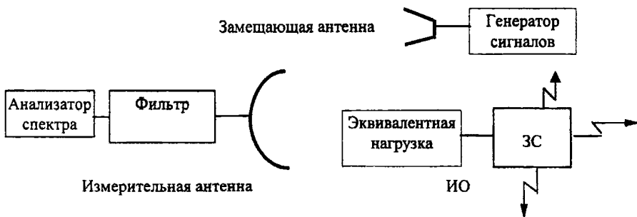
Рисунок 3 - Структурная схема измерения побочных излучений для диапазона частот свыше 1 000 МГц для измерительного оборудования без антенны
