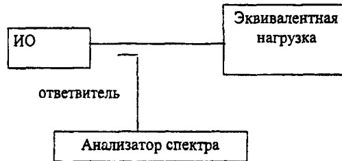
Рисунок 6 - Структурная схема измерения плотности передаваемой выходной мощности
