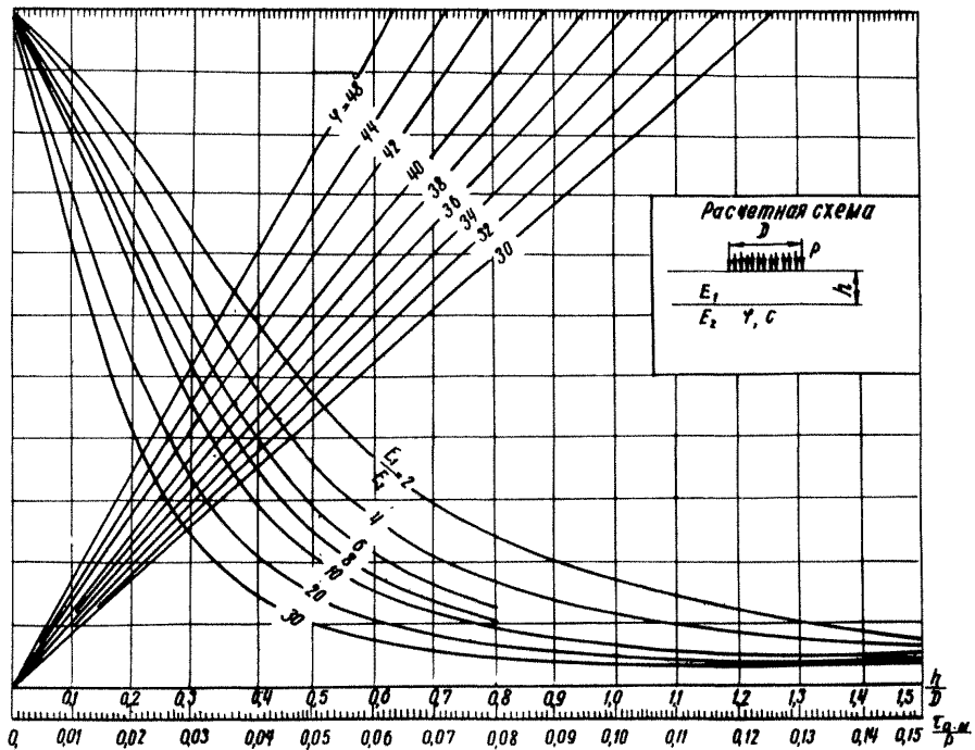
Рис.2. Номограмма для определения активных напряжений сдвига от временной нагрузки \tau_{\alpha, м} в нижнем слое двухслойной системы при свободном смещении слоев на контакте
