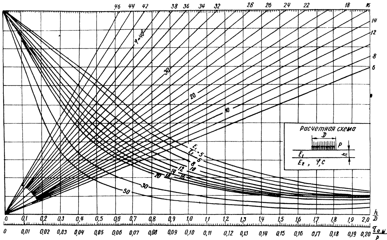
Рис.1. Номограмма для определения активных напряжений сдвига от временной нагрузки \tau_{a.m} в нижнем слое двухслойной системы при совместной работе слоев
