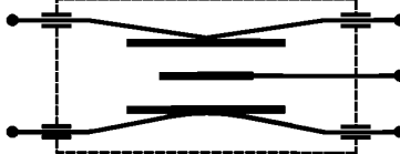
Рисунок 4d — Многосекционный проходной конденсатор
