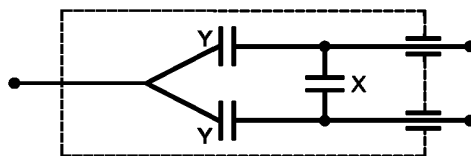
Рисунок 5b — Шунтирующий конденсатор, соединенный по схеме треугольника
