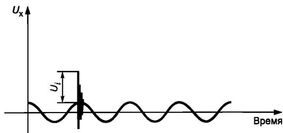
Рисунок 8 — Основная волна переменного напряжения со случайным несинхронизированно наложенным высоковольтным импульсом
