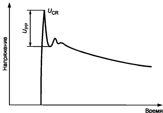
Рисунок 6 — Форма импульса
