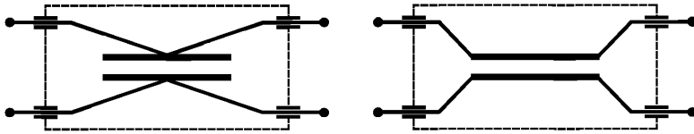
Рисунок 4a — Проходной конденсатор для симметричного включения в цепь (некоаксиальный)
