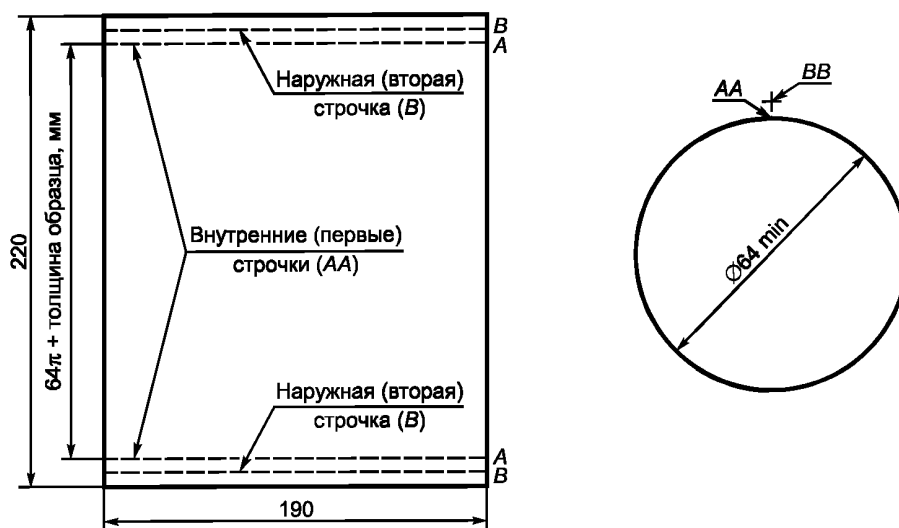
а – образец, размеченный для сшивания
