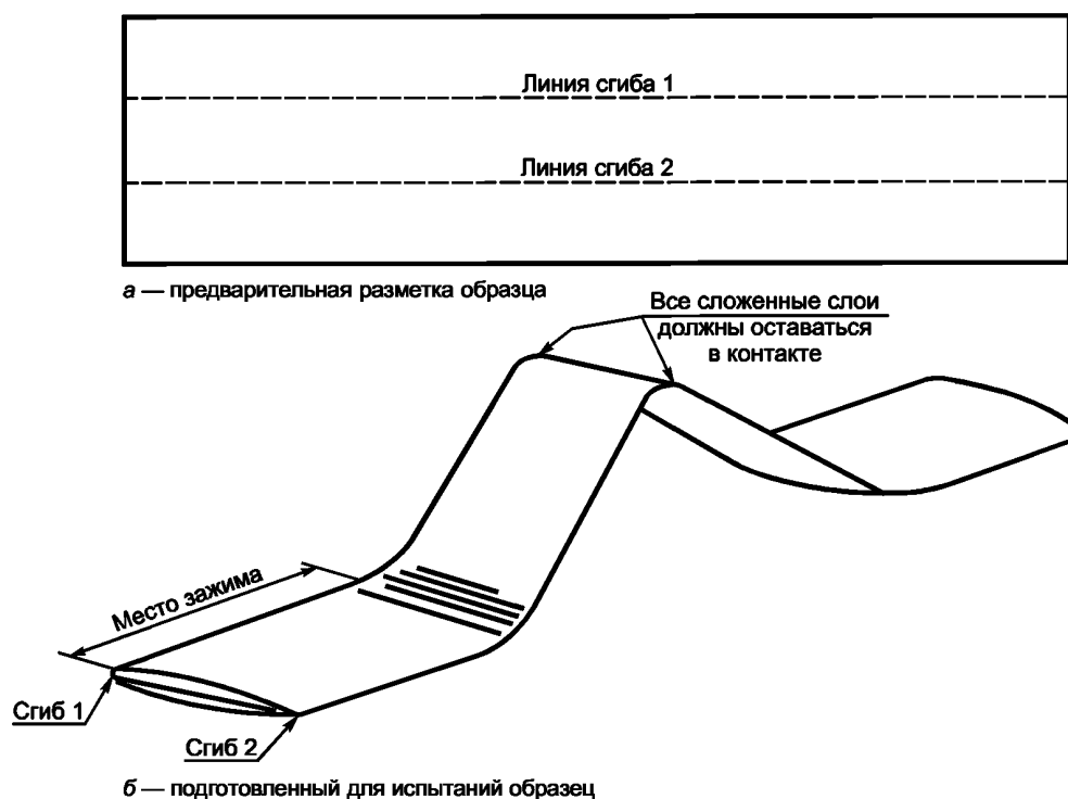
Рисунок 1.1 — Схема складывания и форма образца для испытания по методу Де Маттиа
