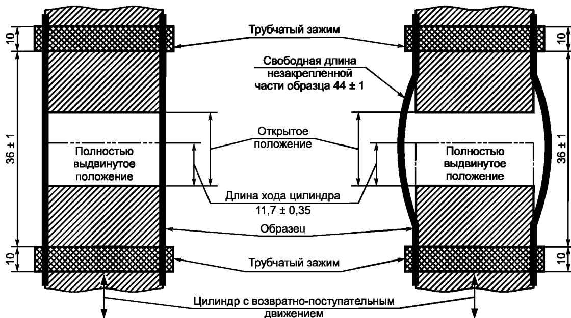
а - стандартный испытуемый образец 105 \times 50 мм
