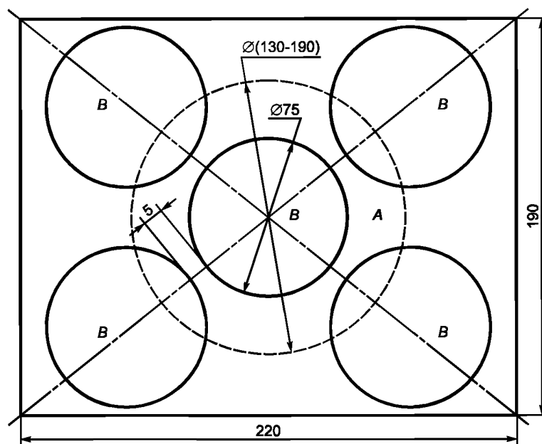
A — для метода А по ИСО 1420; B — для метода В по ИСО 1420
