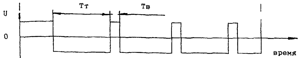
б) Однократная переполюсовка напряжения при ответе вызываемого абонента с много- кратным восстановлением исходной поляр- ности напряжения при тарификации
