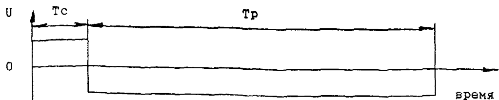
а) Однократная переполюсовка напряжения станционной батареи при ответе вызываемо- го абонента
