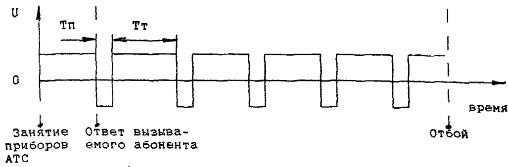
в) многократная переполюсовка напряжения при тарификации
