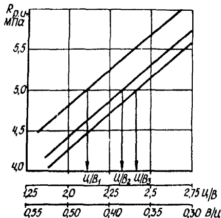
Рис.2. Зависимость прочности R_{p,ц} бетона от Ц/В при различном расходе крупного заполнителя
