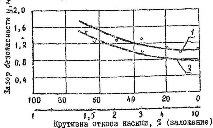
Рис.1. Зависимость зазора безопасности y от крутизны откоса насыпи при движении: 1- на спуск; 2- на подъем
