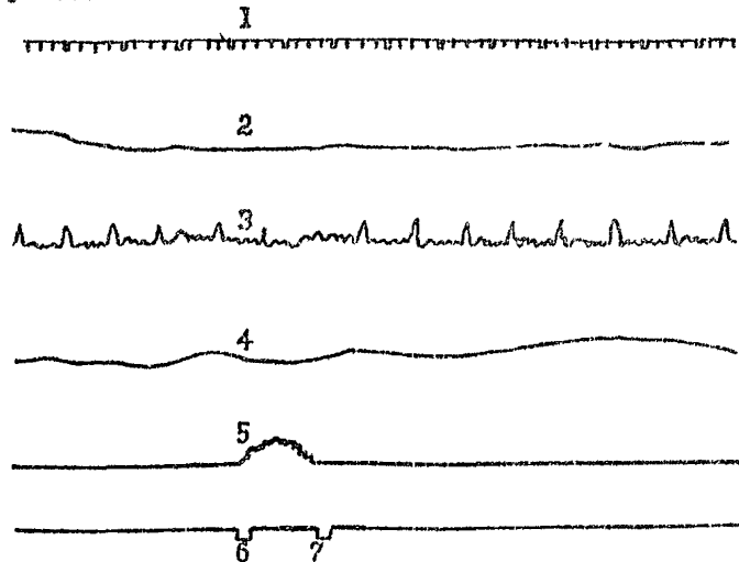
Рис. 1. Психофизиологические показатели водителя и режимы движения на участке смены полосы движения: 1- путь; 2- скорость; 3- ЭКГ; 4- КГР; 5- поперечное ускорение; 6 и 7- соответственно начало и конец маневрирования автомобиля
