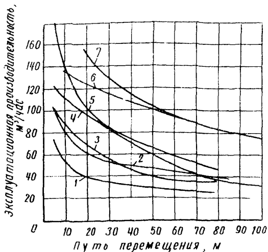
Рис.3. Зависимость эксплуатационной производительности фронтальных погрузчиков по маркам от длины транспортного пути: 1-Д-561; 2-ТО-17; 3-Т-157; 4-Т-157 (экспериментальные данные); 5-Д-543; 6-Д-660; 7-Д-660 (экспериментальные данные)
