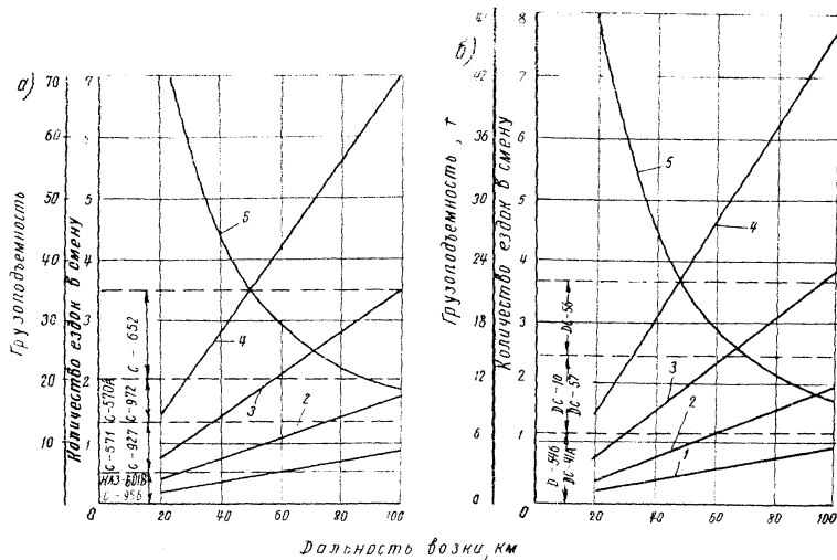
Рис.2. Влияние дальности возки на выбор грузоподъемности цементовозов (а) и битумовозов (б) в зависимости от производительности АБЗ: 1-П=25 т/час; 2-П=50 т/час; 3-П=100 т/час; 4-П=200 т/час; 5-количество ездов
