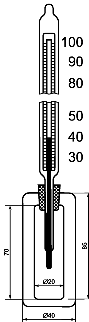
Рисунок 1 — «Прибор Жукова»
