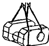
Схема строповки детали прессы
