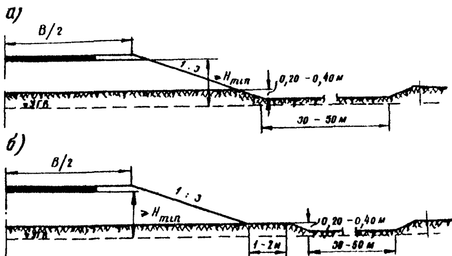
Рис.1. Конструкция земляного полотна на мокрых солончаках I типа: а - при наличии верхнего сухого слоя грунта или возможности естественного его осушения; б - при невозможности отвода воды из резерва
