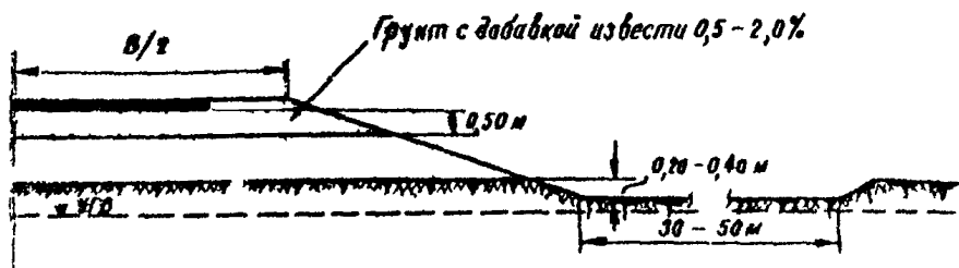
Рис.2. Конструкция земляного полотна на мокрых солончаках при влажности выше оптимальной и невозможности естественного осушения грунта
