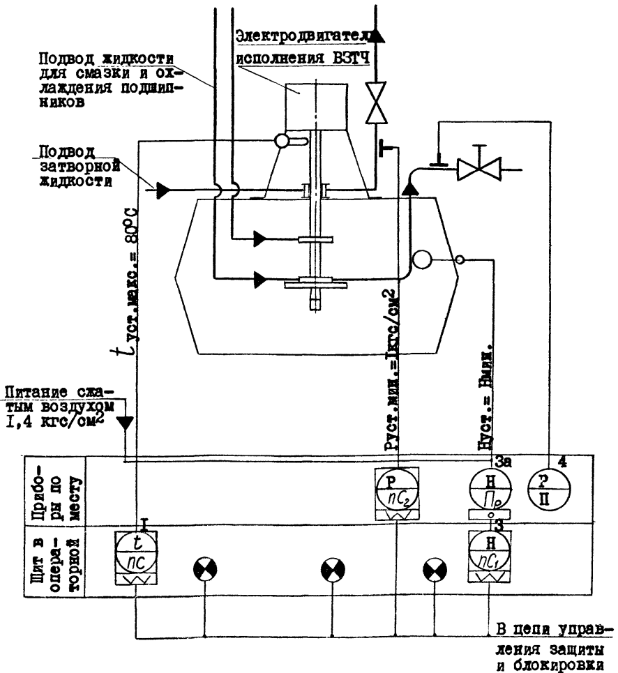
Схема защиты, блокировки и сигнализации насосного агрегата.
