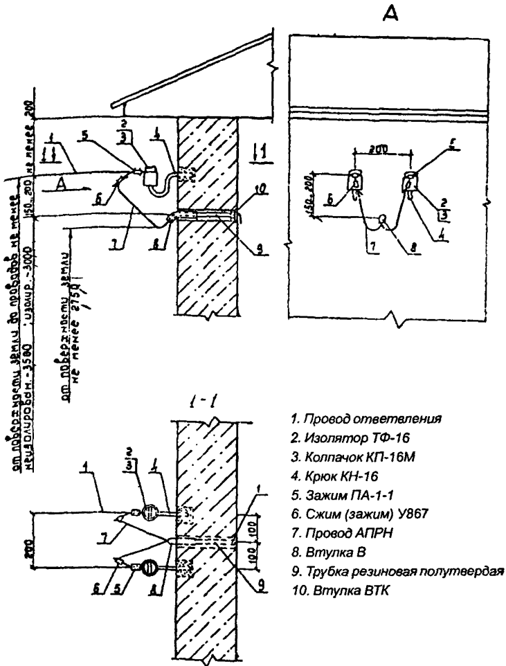
Рис. 2.2.2. Устройство воздушного ввода от ВЛ неизолрированным (изолированным) проводом, стены кирпичные (бетонные).
