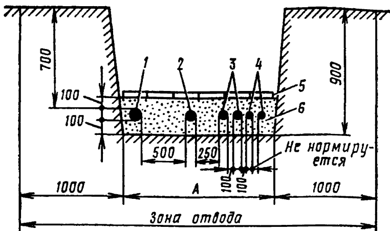
Рис. 3.2.3. Минимальные расстояния между кабелями, прокладываемыми в траншеях:
