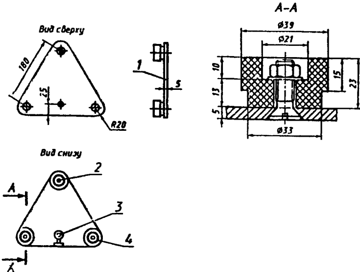
Рис. А.1. Испытательный электрод 2
