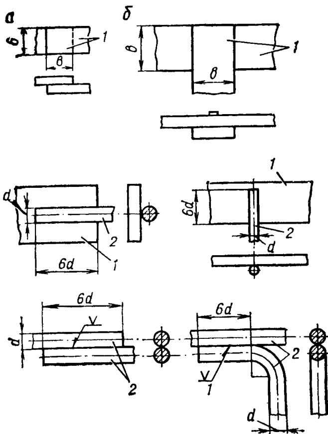
Рис. 3.1.5. Сварные соединения заземляющих проводников: a — продольные соединения; б — ответвления: 1 — проводник из полосовой стали; 2 — проводник из круглой стали.
