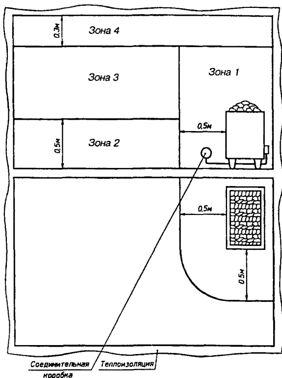
Рис. 2.2.10. Зоны температур в помещениях саун (согласно ГОСТ Р 50571.12.96)
