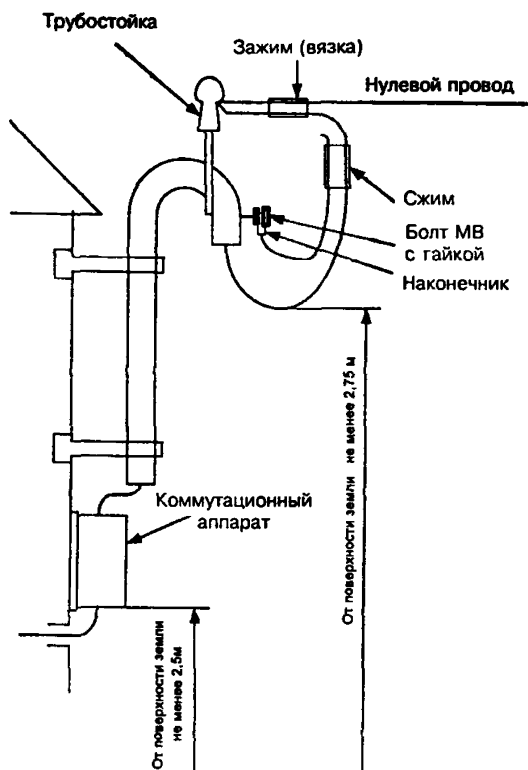
Рис. 2.3.3. Устройство ввода в здание через трубостойку.
