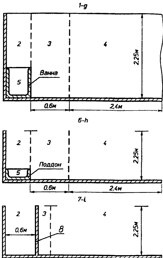
Рис. 2.2.9.6. Зоны в ваннных и душевых помещениях, вертикальный разрез (согласно ГОСТ Р-50571.11.96.):
