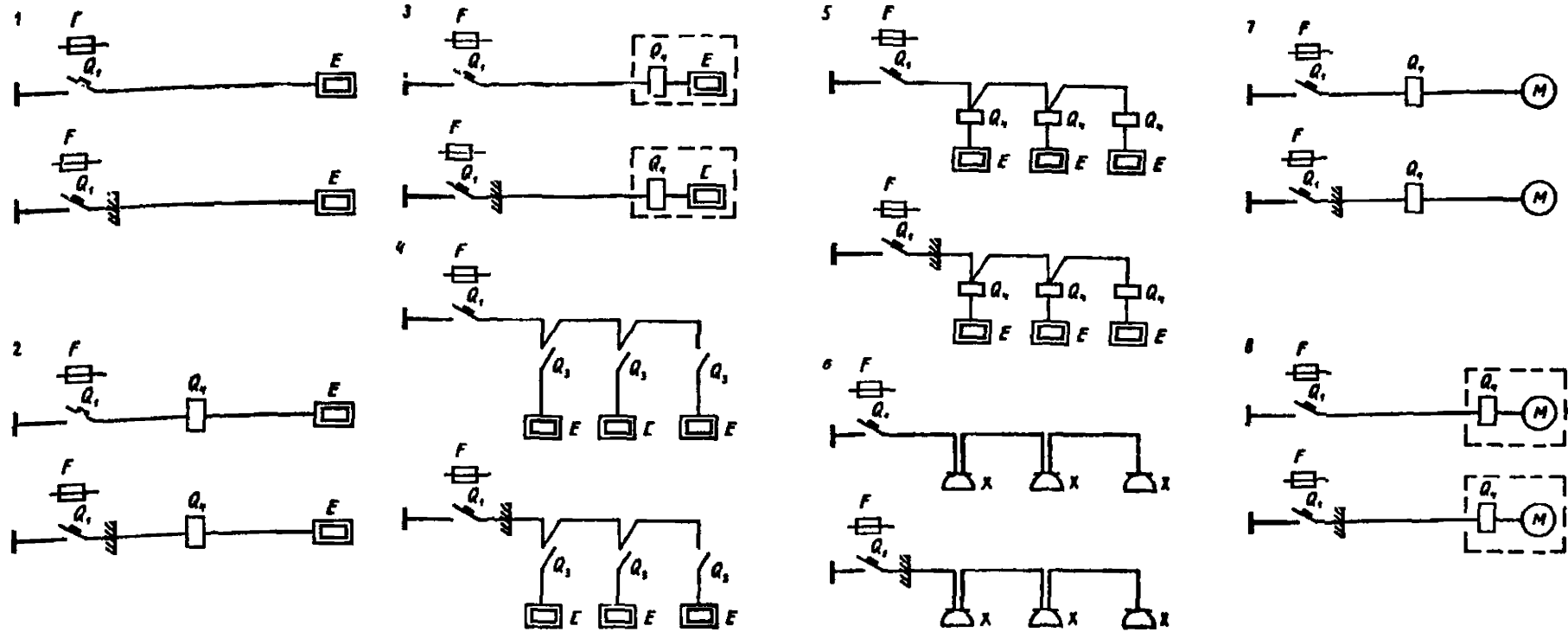
Рис. 2.4.2 (1—8). Схемы присоединения силовых электроприемников технологического (теплового или механического) оборудования: \vdash — распределительный пункт (РП), Q_1 — автоматический выключатель, устанавливаемый в РП; F_1 — предохранитель; Q_2 — автоматический выключатель; K — магнитный пускатель; S — выключатель в цепи управления; Q_3 — выключатель в главной цепи; M — механический или холодильный токоприемник; E — тепловой токоприемник; X — электрический соединитель в защитном исполнении с заземляющим контактом; Q_4 — коммутационный аппарат (пускатель, рубильник и т. п.) может поставляться комплектно с оборудованием; «—» — перегородка.
