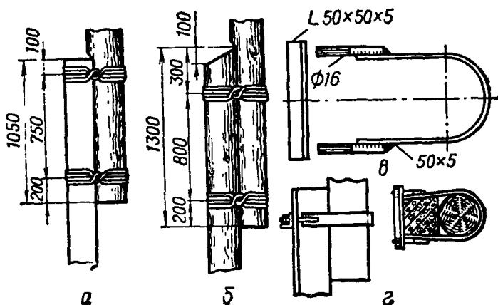
Рис. 3.3.3. Соединение стойки опор ВЛ 0,4 кВ с приставкой: а — железобетонной; б — деревянной; в — хомут для соединения деревянных стоек с железобетонной приставкой; г — готовое соединение хомутом.
