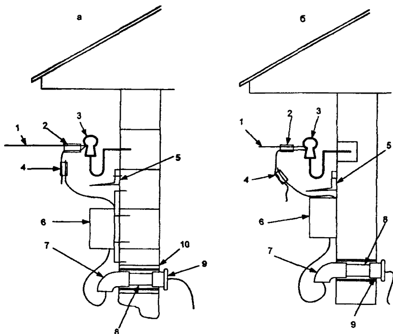
Рис. 2.3.2. Устройство ввода в здание: а — стены деревянные; б — стены кирпичные (бетонные); 1 — провод ответвления; 2 — зажим (вязка); 3 — изолятор ТФ-12; 4 — сжим; 5 — защитный козырек; 6 — коммутационный аппарат; 7 — втулка типа В; 8 — трубка резиновая (полутвердая); 9 — втулка типа ВТК; 10 — труба стальная.
