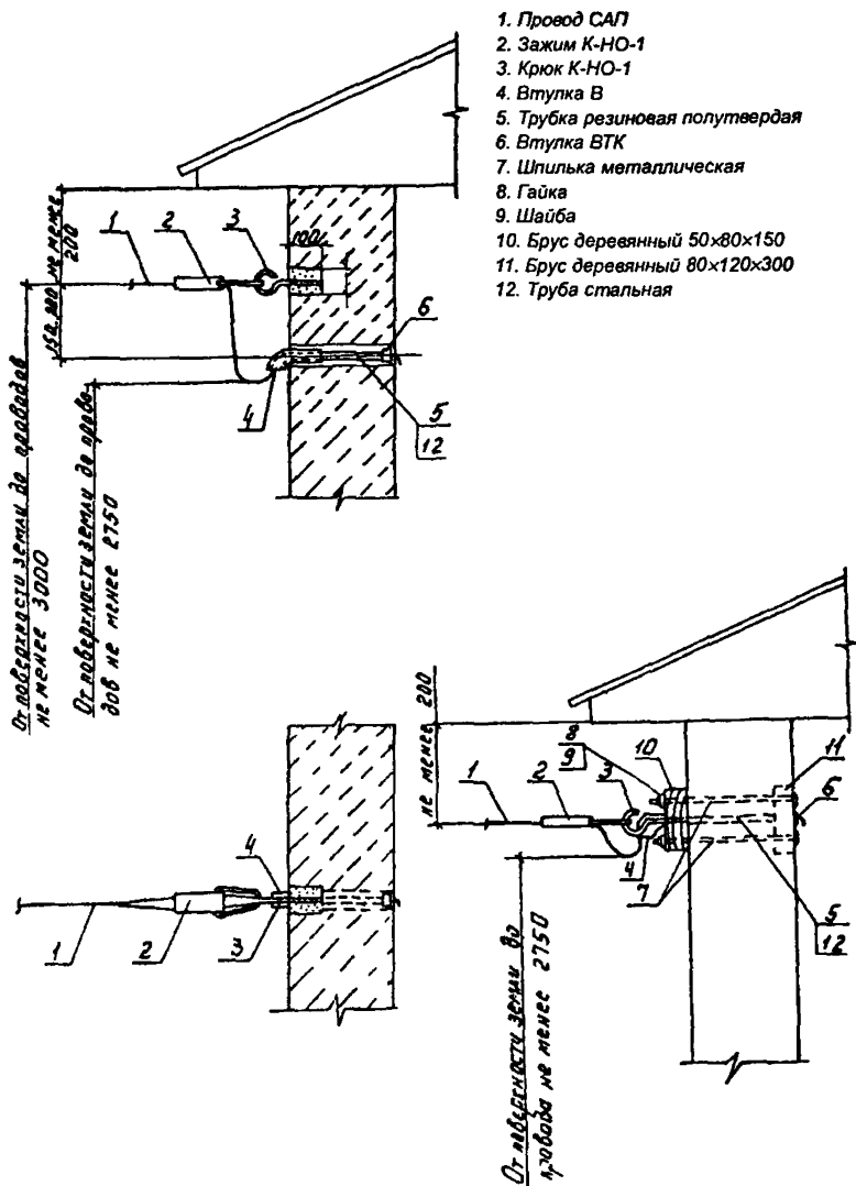
Рис. 2.2.4. Устройство воздушного ввода от ВЛ самонесущим проводом. Стены кирпичные (бетонные).
