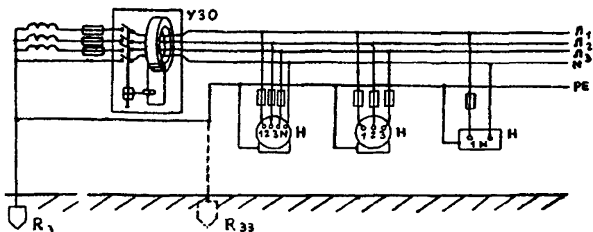
Рис. 2.2.7. Схема установки УЗО в четырехпроводной сети с глухозаземленной нейтралью в системе TN-S (нулевой рабочий N и нулевой защитный PE проводники разъединены): L1, L2, L3 — линейные проводники; H — нагрузка; R_3 — рабочее заземление; R_{33} — защитное заземление
