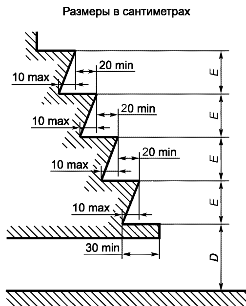
Рисунок Г.4 — Ступеньки для пассажиров (см. 5.7.7)
