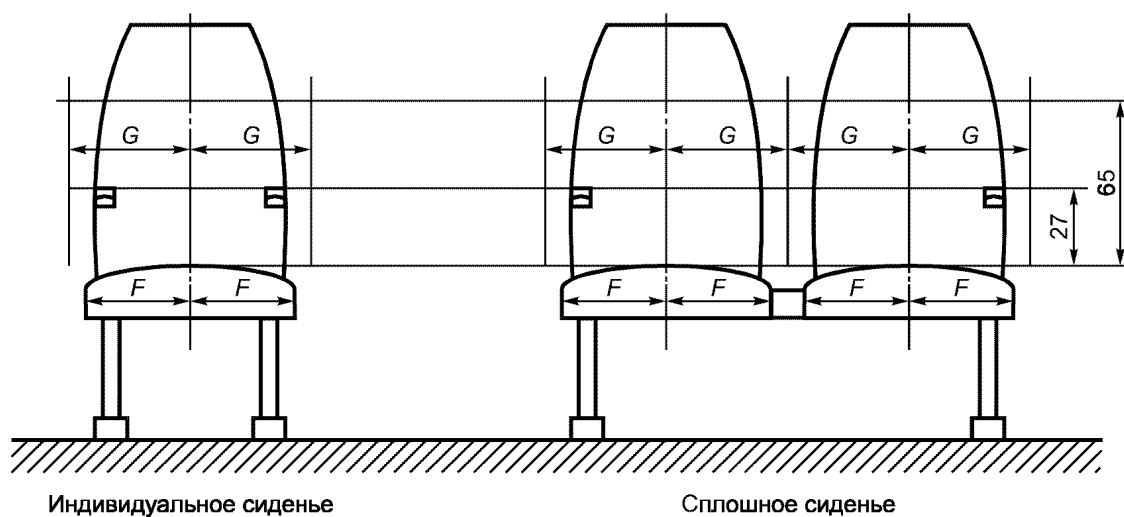
Рисунок Г.5 — Ширина пассажирских сидений (см. 5.7.8.1)
