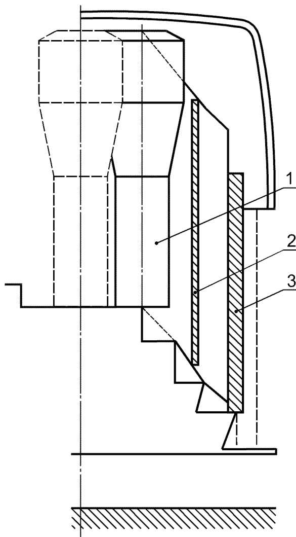
1 — цилиндрический шаблон; 2 — вертикальный шаблон; 3 — двойной шаблон
