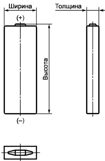
Рисунок 2 — Малогабаритный призматический аккумулятор
