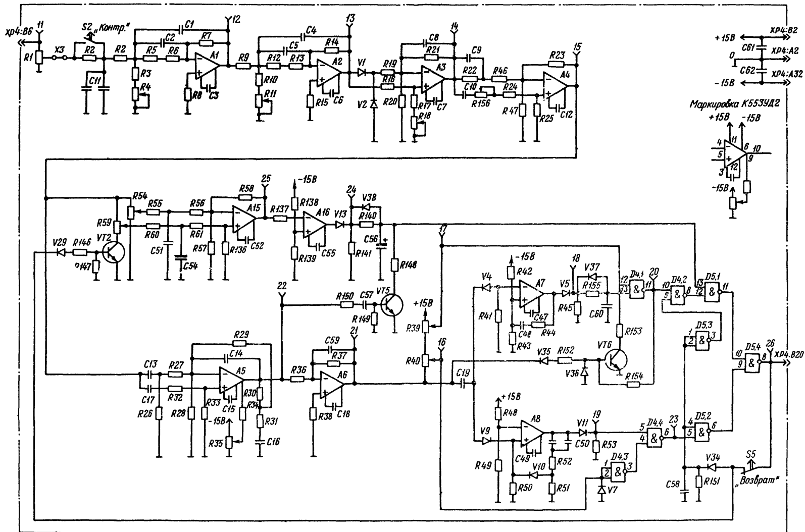
Рис.5. Принципиальная электрическая схема БТГ блока защиты БФ0 1301.02
