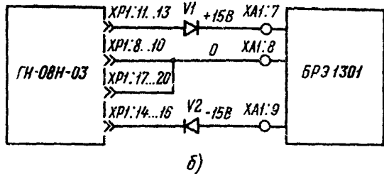
Рис.П7.1. Схема включения источника питания ГН-08Н-03: а - цепи постоянного оперативного тока; б - выходные цепи при использовании для питания блока защиты БРЭ 1301 второго и третьего каналов
