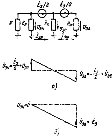
Рис. ПЗ.3. Эквивалентная схема замещения сети генераторного напряжения блока генератор-трансформатор для оставшихся третьей гармоники:
