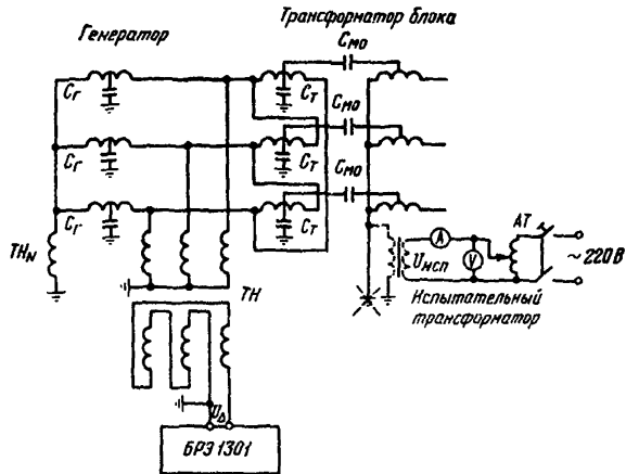
Рис. ПБ.1. Схема энергоблока при проведении измерений, необходимых для расчета уставки БОС
