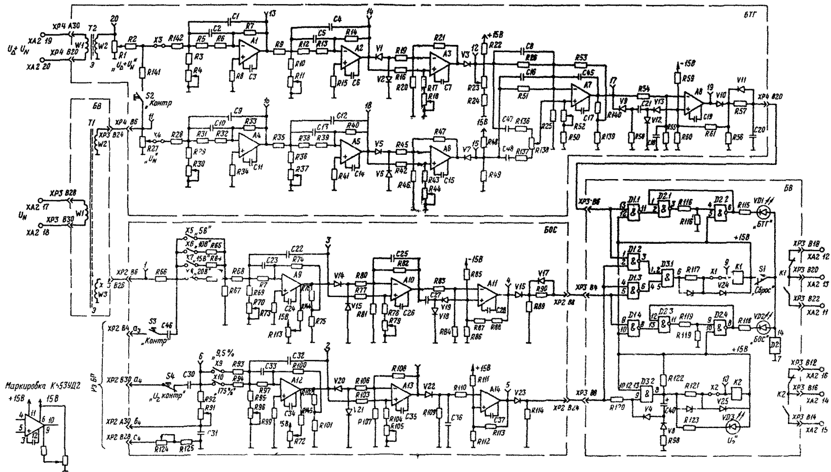
Рис.3. Принципиальная электрическая схема блока защиты БРЭ 1301.01
