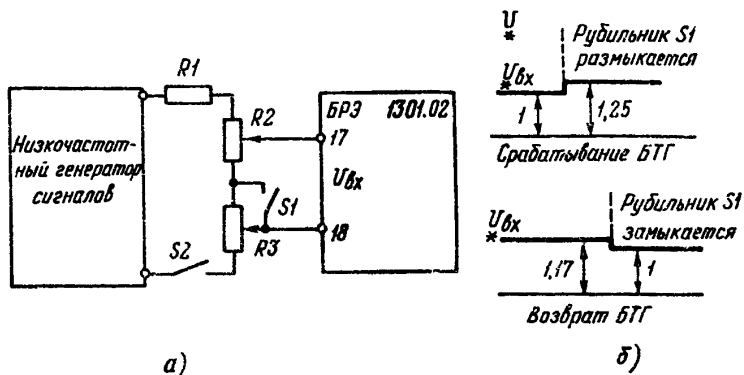
Рис.6. Схема проверки БТГ блока защиты БРЭ I301.02:
