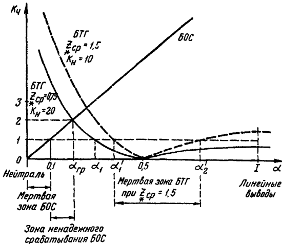
Рис. П2.4. График зависимости коэффициента чувствительности БТГ и БОС блока защиты БРЭ 1301.01 от относительного количества витков обмотки статора от нейтрали до места замыкания для энергоблоков 300 МВт при Z_{*cp}^* = 15 и U_{cp,BOC} = 10 В; \alpha_1 = 0,3 ; \alpha'_1 = 0,37 ; \alpha'_2 = 0,75
