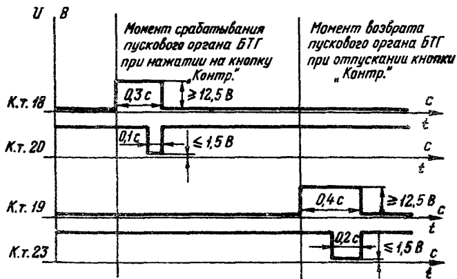
Рис.7. Временная диаграмма работы пускового органа БТГ блока защиты БРЗ 1301.02 при его срабатывании и возврате от кнопки "Контр."
