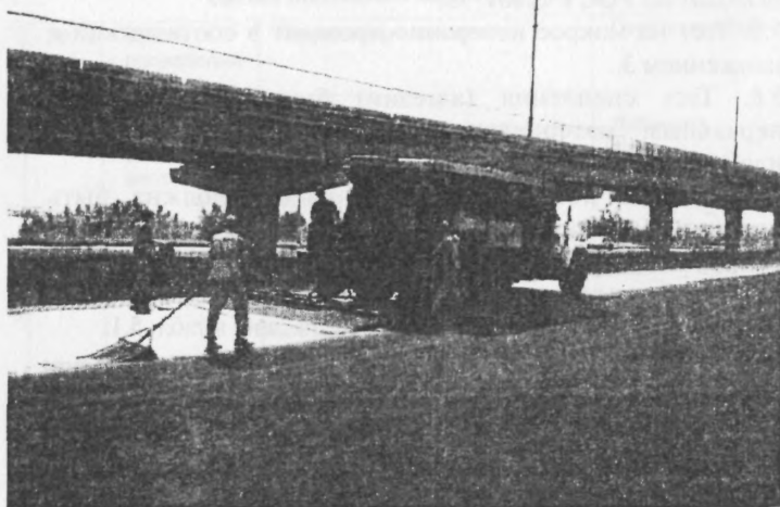
Рис. 4.3. Устройство слоя износа «Сларри Сил» на улицах г. Воронежа
