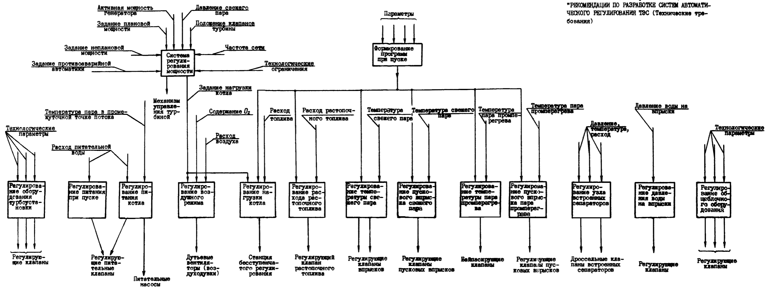
Обобщенная структурная схема АР энергоблока с прямоточным котлом
