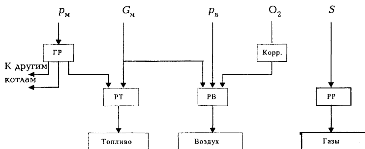
Рис. 1. Типовая схема регулирования нагрузки барабанного котла:
