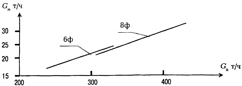
Рис. 2. Статические характеристики давления мазута ( p_m ), перепада давлений "воздух - топка" ( \Delta p_{вт} ) и расхода мазута ( G_m ) когда БКЗ-420-140 при работе на шести и восьми форсунках (ф)
