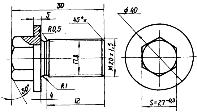
Рис. 3-1-3. Пробка
