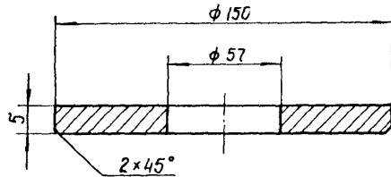
Рис.3-1-1. Дно
