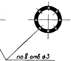
Рис. 2-5-2. Корпус
