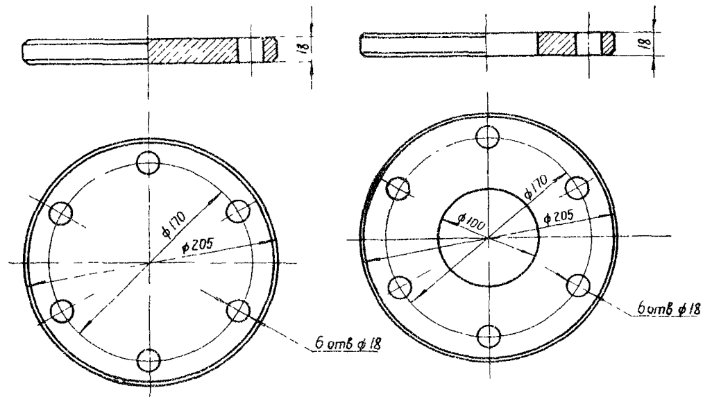
Рис. 5-I-2. Фланец
