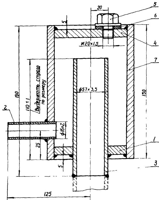
Рис.3-1. Конденсационный сосуд для измерения низких давлений:
