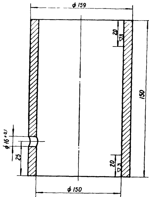
Рис. 3-1-4. Стакан
