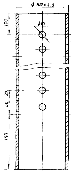
Рис. 5-I-3. Труба
