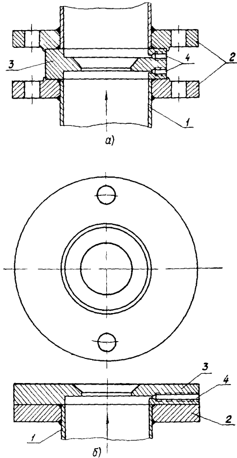
Рис. 14. Устройство для измерения расхода воздуха, удаляемого пароструйным эжектором: а - отвод паровоздушной смеси в атмосферную трубу; б - отвод паровоздушной смеси в машинный зал: 1 - выхлопная труба; 2 - фланец; 3 - измерительная диафрагма; 4 - точка отбора импульса
