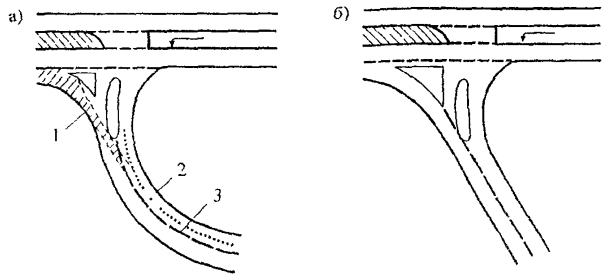
Рис. 8.7. Зрительное перекрытие островками неправильного направления движения:
