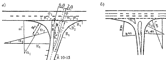
Рис. 8.10. Расположение островков на второстепенной дороге: а – схема размещения островка; б – выделение островка разметкой
