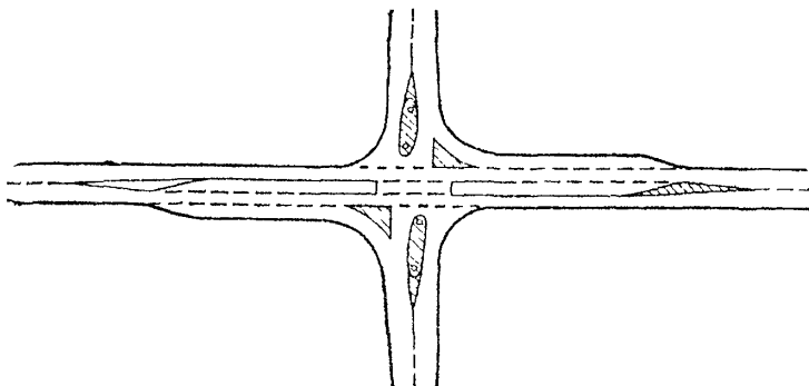
Рис. 8.13. Выделение островков на проезжей части разметкой
