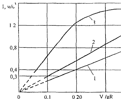
Рис. 4.2. График для определения расчетного нарастания центробежного ускорения
