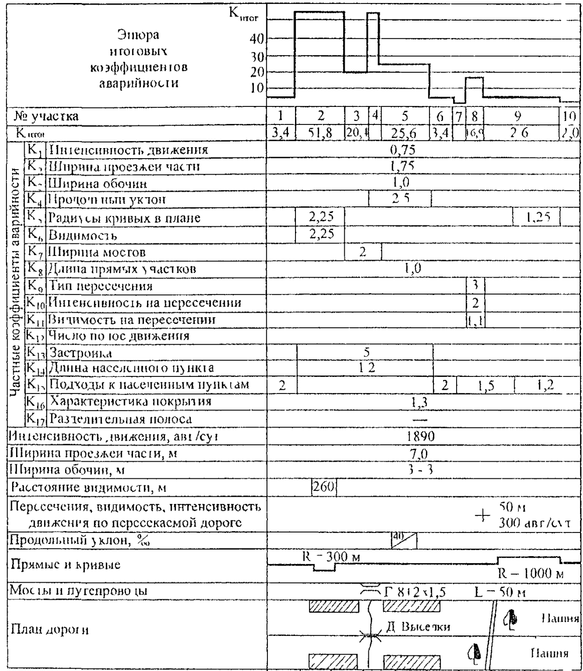
Рис. 1.2. Пример графика итогового коэффициента аварийности 1.4.8.
