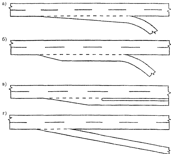
Рис. 9.2. Типы переходно-скоростных полос
