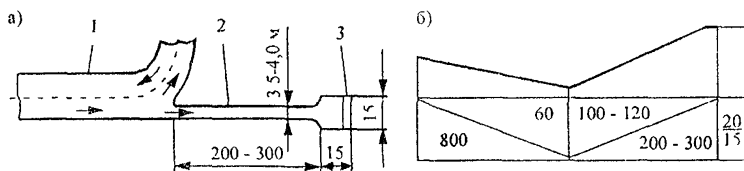
Рис. 5.1. Схема аварийного съезда: а – план; б – продольный профиль; 1 – основная дорога; 2 – аварийный съезд; 3 – песчаный вал
