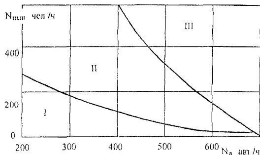
Рис. 11.2. Области применения пешеходных переходов различных типов: I – нерегулируемые переходы; II – светофорное регулирование; III – внеуличные пешеходные переходы
