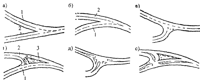
Рис. 8.5. Рекомендуемые схемы планировки пересечений в одном уровне на обходе населенных пунктов: а, б – неправильная схема без разделения дорог на главную и второстепенную; в, з – рекомендуемые схемы при невысокой интенсивности движения на второстепенной дороге; д, е – то же, при высокой интенсивности; 1 – главная дорога; 2 – второстепенная дорога; 3 – распределительная полоса
