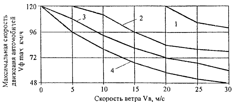
Рис. 1.3. Зависимости максимальной безопасной скорости движения автомобилей от скорости ветра:
