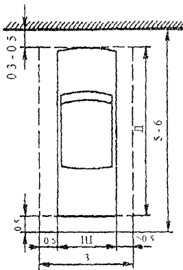
Рис. 11.4. Размеры (м) ячейки для хранения автомобиля на стоянках: Д и Ш - габаритные длина и ширина расчетного автомобиля, соответственно
