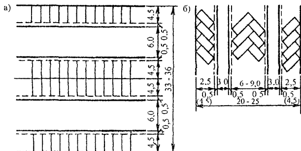
Рис. 11.8. Размеры планировочных элементов (м) стоянок с многорядной расстановкой автомобилей: а - под прямым углом; б - под острым углом
