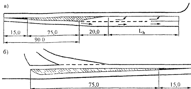
Рис. 8.11. Расположение островков на главной дороге: а – левоворотный островок; б – направляющий островок
