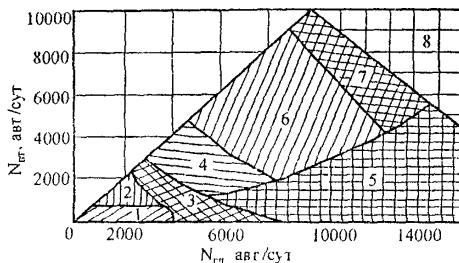
Рис. 8.1. Номограмма для выбора типа планировочных решений пересечений:
