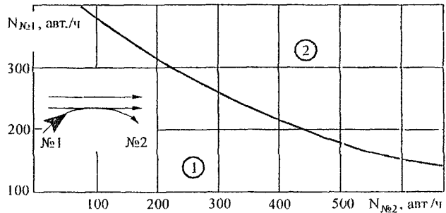
Рис. 9.3. Диаграмма применимости различных типов левоповоротных съездов:
