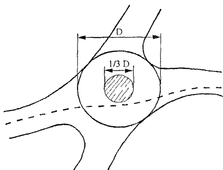
Рис. 8.15. Улучшение условий движения на пересечении путем устройства островков небольшого диаметра
