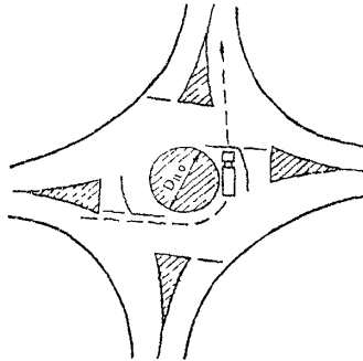
Рис. 8.17. Схема расположения автоезда в зоне ожидания на кольцевой проезжей части
