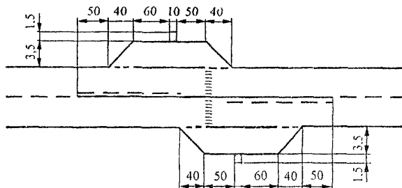
Рис. 11.9. Планировка автобусных остановок в населенных пунктах
