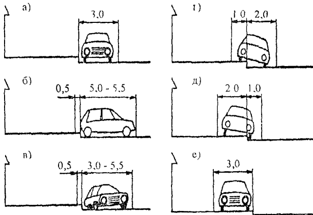
Рис. 11.6. Размещение стоянок в пределах улицы: а - расстановка автомобилей вдоль улицы; б - поперечная расстановка; в - расстановка под углом; г-д - частичное использование тротуара; е - расстановка на тротуаре
