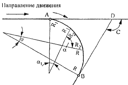
Рис. 8.3. Схема для расчета коробовой кривой
