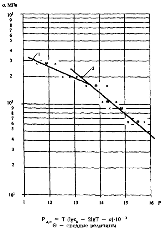
Рисунок 2 – Условная параметрическая диаграмма длительной прочности
