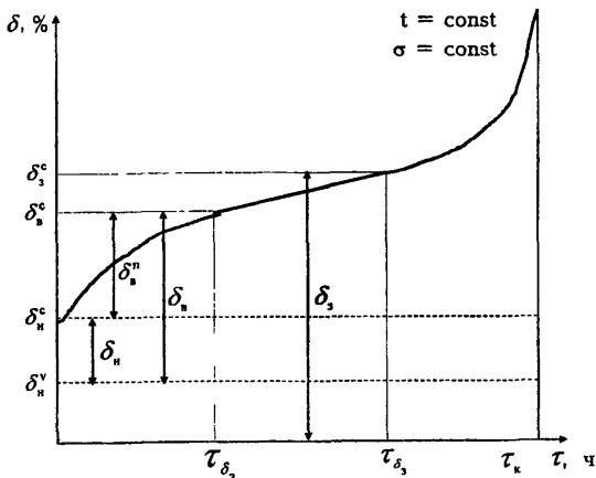
Рисунок 1 – Кривая деформирования
