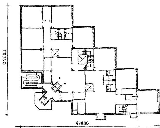
Рис. 8 Проект блока-пристройки на 8 начальных классов 200 учащихся И-1745/2А (разработан в 1998 году). Фасады и план первого этажа.
