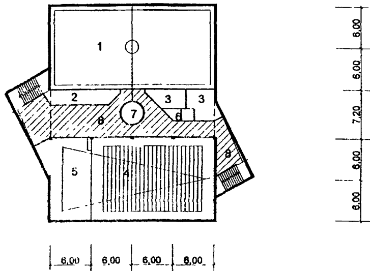
Рис 29 Схема архитектурно-планировочного решения блока общешкольных помещений с залами «БОП-1»
