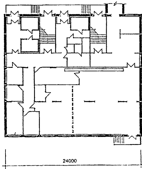
План 1 этажа
