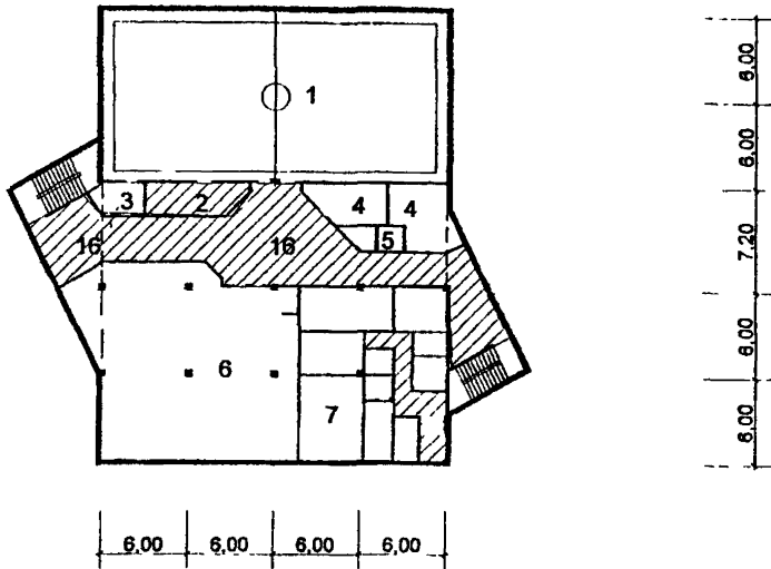
Рис. 28 Схема архитектурно-планировочного решения блока общешкольных помещений с залами «БОП-1»
