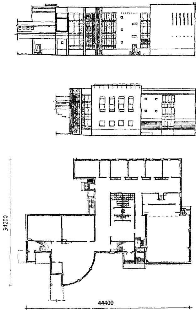
Рис.9 Проект блока-пристройки специализированных учебных кабинетов на 250 учащихся (разработан в 2003г.) И-2025. Фасады и план I этажа.
