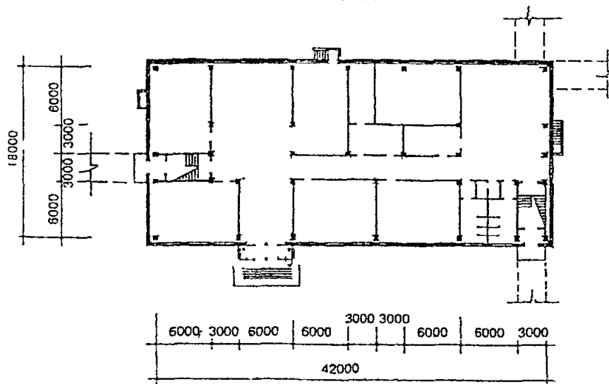
План 1 этажа
